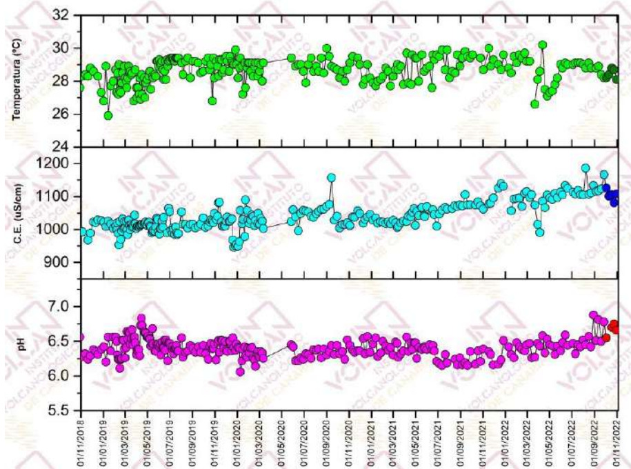
Figura 4.9 - Variaciones temporales de temperatura, conductividad ( \mu\text{S}\cdot\text{cm}^{-1} ) y pH medidas en el agua subterránea de la estación geoquímica TFG03. Los datos de octubre de 2022 se encuentran indicados en diferentes colores.
