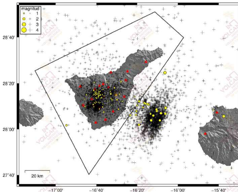
Figura 1.1 - Hipocentros de los terremotos (círculos amarillos) localizados por las estaciones de la Red Sísmica Canaria (triángulos rojos) en octubre de 2022. Las cruces muestran los hipocentros localizados en los últimos 12 meses. El polígono negro corresponde al área de Tenerife considerada en las estadísticas sismológicas de los gráficos siguientes.
