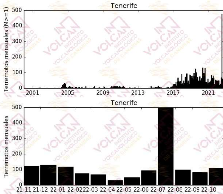
Figura 1.2 - Número de terremotos mensuales en Tenerife. El histograma superior corresponde al periodo enero 2001 – octubre 2022 para terremotos con M \geq 1 , mientras que el inferior muestra el periodo noviembre 2021 – octubre 2022 para todas las magnitudes. [La fuente de los datos sísmicos anteriores al 21/11/2016 es el Instituto Geográfico Nacional, IGN].
