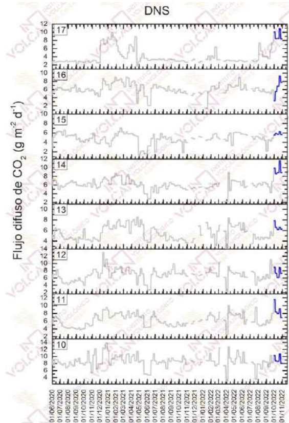
Figura 4.6 – Monitorización semanal del flujo difuso de CO 2 en la Red de Trampas Alcalinas del sistema volcánico Dorsal Norte-Sur de Tenerife desde junio de 2020. Los datos de octubre de 2022 se encuentran indicados en azul oscuro.
