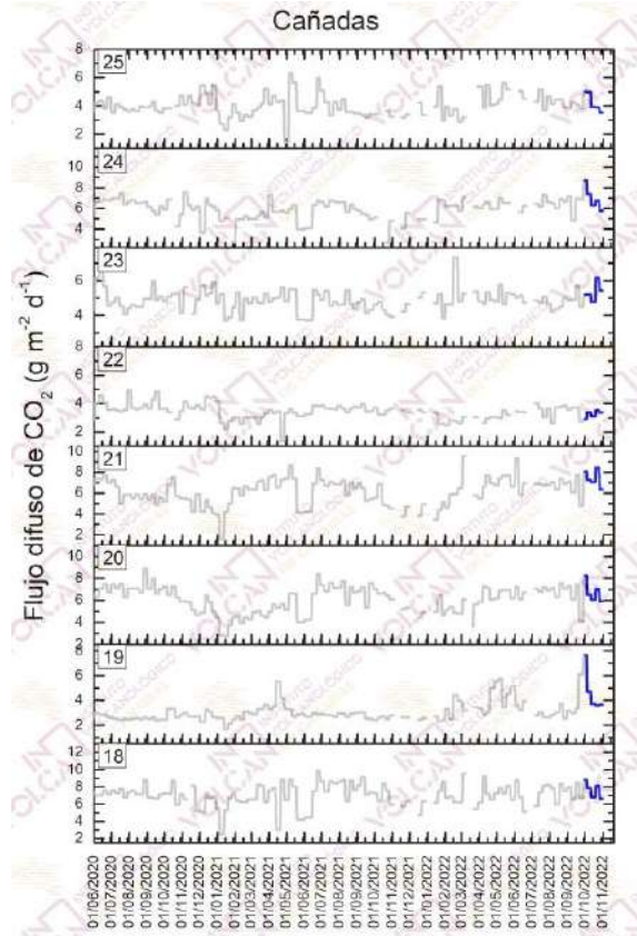
Figura 4.7 – Monitorización semanal del flujo difuso de CO 2 en la Red de Trampas Alcalinas de la Caldera de Las Cañadas desde junio de 2020. Los datos de octubre de 2022 se encuentran indicados en azul oscuro.
