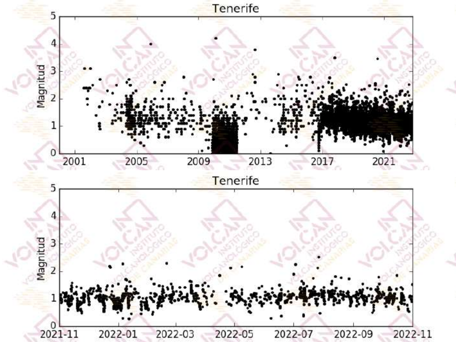
Figura 1.4 - Magnitudes de los terremotos localizados en el área de Tenerife. El gráfico superior corresponde al periodo enero 2001 – octubre 2022, mientras que el inferior muestra el periodo noviembre 2021 – octubre 2022. [La fuente de los datos sísmicos anteriores al 21/11/2016 es el Instituto Geográfico Nacional, IGN].
