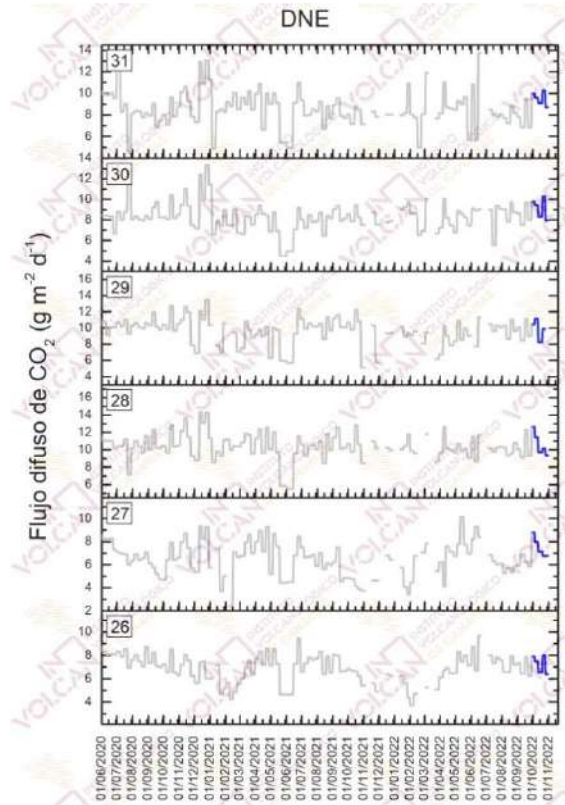
Figura 4.5 – Monitorización semanal del flujo difuso de CO 2 en la Red de Trampas Alcalinas del sistema volcánico Dorsal Noreste de Tenerife desde junio de 2020. Los datos de octubre de 2022 se encuentran indicados en azul oscuro.
