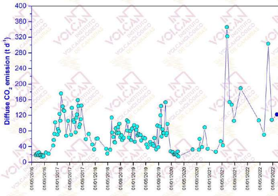
Figura 4.3 – Variaciones temporales de la emisión difusa de dióxido de carbono (CO 2 ) en el cráter del Teide desde el 1 de mayo de 2016 hasta octubre 2022. Los datos de octubre de 2022 se encuentran indicados en azul oscuro.
