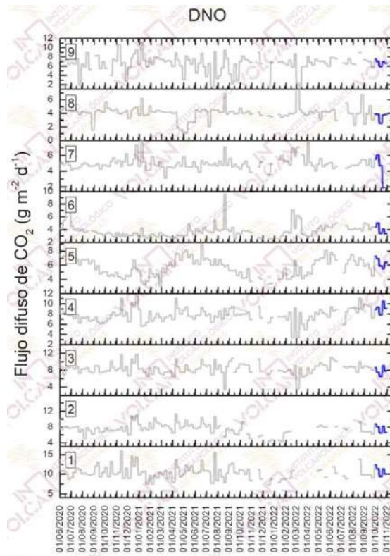
Figura 4.4 – Monitorización semanal del flujo difuso de CO 2 en la Red de Trampas Alcalinas del sistema volcánico Dorsal Noroeste de Tenerife desde junio de 2020. Los datos de octubre de 2022 se encuentran indicados en azul oscuro.
