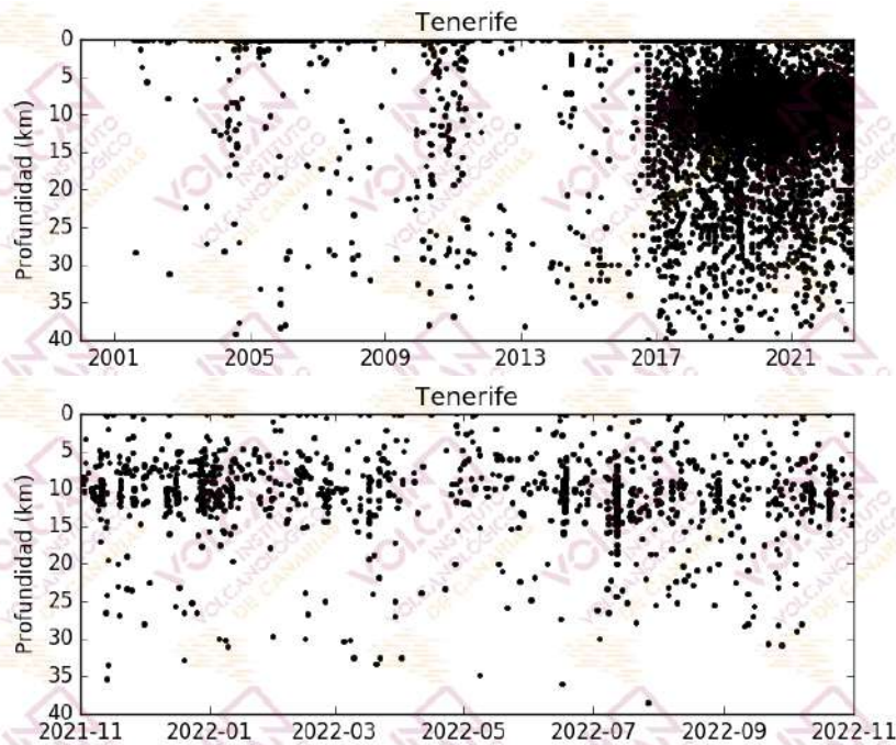
Figura 1.3 - Profundidades de los hipocentros localizados en el área de Tenerife. El gráfico superior corresponde al periodo enero 2001 - octubre 2022, mientras que el inferior muestra el periodo noviembre 2021 – octubre 2022. [La fuente de los datos sísmicos anteriores al 21/11/2016 es el Instituto Geográfico Nacional, IGN].
