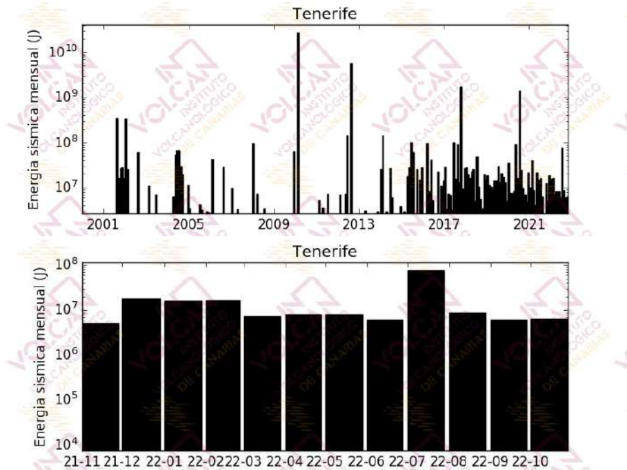
Figura 1.5 – Energía sísmica liberada por los terremotos localizados en el área de Tenerife. El histograma superior corresponde al periodo enero 2001 – octubre 2022, mientras que el inferior muestra el periodo noviembre 2021 – octubre 2022. [La fuente de los datos sísmicos anteriores al 21/11/2016 es el Instituto Geográfico Nacional].
