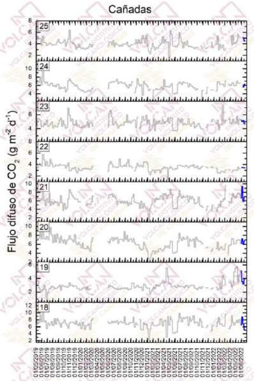
Figura 4.7 – Monitorización semanal del flujo difuso de CO 2 en la Red de Trampas Alcalinas de la Caldera de Las Cañadas desde mayo de 2019. Los datos de junio de 2022 se encuentran indicados en azul oscuro.
