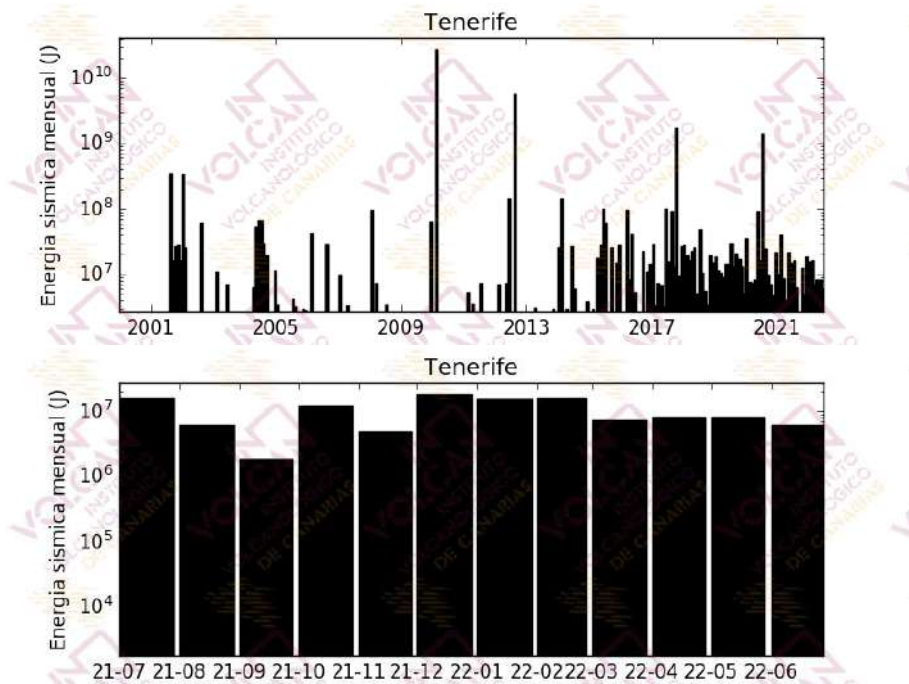
Figura 1.5 – Energía sísmica liberada por los terremotos localizados en el área de Tenerife. El histograma superior corresponde al periodo enero 2001 – junio 2022, mientras que el inferior muestra el periodo julio 2021 – junio 2022. [La fuente de los datos sísmicos anteriores al 21/11/2016 es el Instituto Geográfico Nacional].
