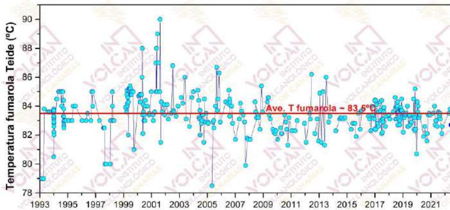
Figura 2.1 – Variaciones temporales de la temperatura registrada en las fumarolas del Teide (TEF1) desde 1993 hasta junio 2022.
