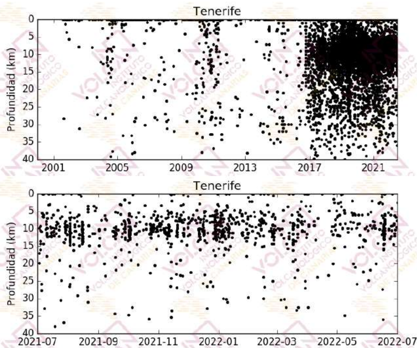
Figura 1.3 - Profundidades de los hipocentros localizados en el área de Tenerife. El gráfico superior corresponde al periodo enero 2001 - junio 2022, mientras que el inferior muestra el periodo julio 2021 – junio 2022. [La fuente de los datos sísmicos anteriores al 21/11/2016 es el Instituto Geográfico Nacional, IGN].
