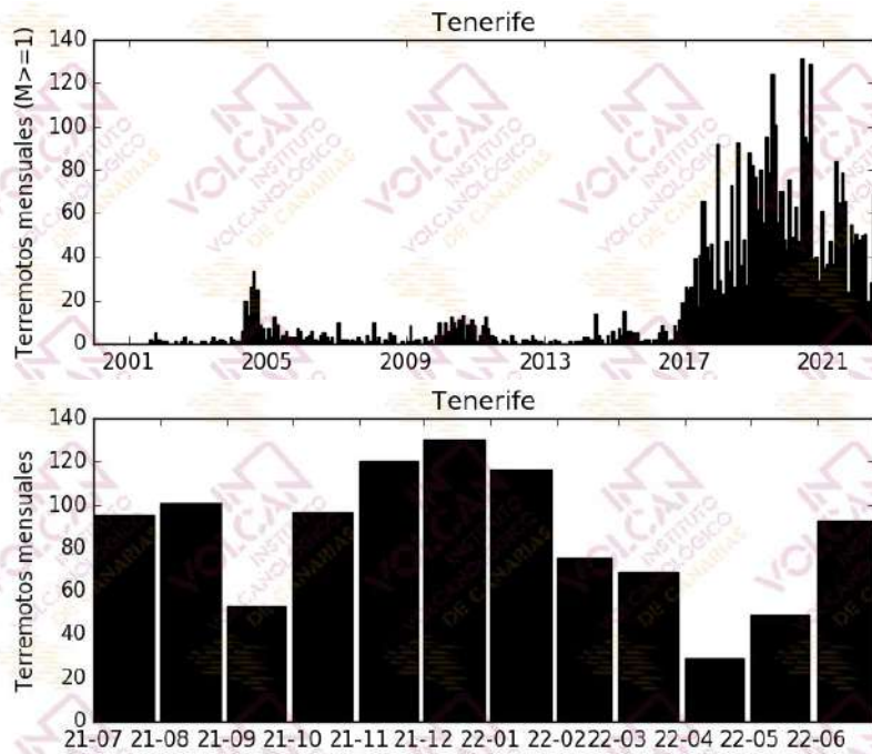
Figura 1.2 - Número de terremotos mensuales en Tenerife. El histograma superior corresponde al periodo enero 2001 – junio 2022 para terremotos con M \geq 1 , mientras que el inferior muestra el periodo julio 2021 – junio 2022 para todas las magnitudes. [La fuente de los datos sísmicos anteriores al 21/11/2016 es el Instituto Geográfico Nacional, IGN].
