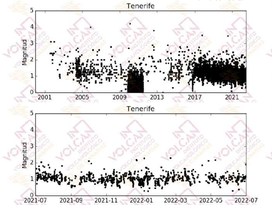
Figura 1.4 - Magnitudes de los terremotos localizados en el área de Tenerife. El gráfico superior corresponde al periodo enero 2001 – junio 2022, mientras que el inferior muestra el periodo julio 2021 – junio 2022. [La fuente de los datos sísmicos anteriores al 21/11/2016 es el Instituto Geográfico Nacional, IGN].
