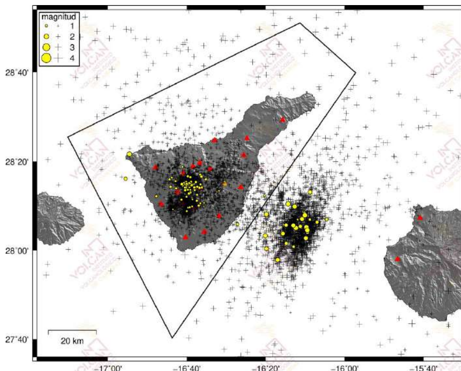
Figura 1.1 - Hipocentros de los terremotos (círculos amarillos) localizados por las estaciones de la Red Sísmica Canaria (triángulos rojos) en junio de 2022. Las cruces muestran los hipocentros localizados en los últimos 12 meses. El polígono negro corresponde al área de Tenerife considerada en las estadísticas sismológicas de los gráficos siguientes.
