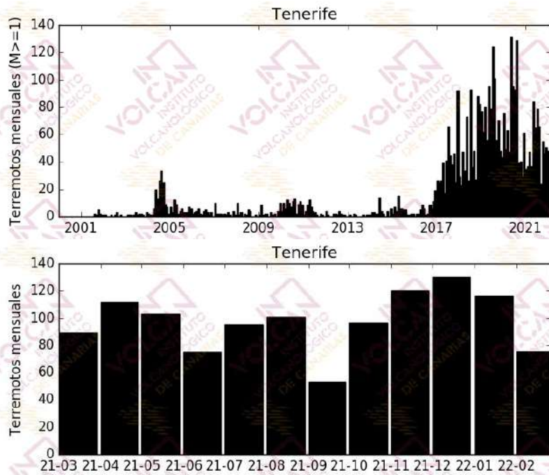
Figura 1.2 - Número de terremotos mensuales en Tenerife. El histograma superior corresponde al periodo enero 2001 – febrero 2022 para terremotos con M \geq 1 , mientras que el inferior muestra el periodo marzo 2021 – febrero 2022 para todas las magnitudes. [La fuente de los datos sísmicos anteriores al 21/11/2016 es el Instituto Geográfico Nacional, IGN].
