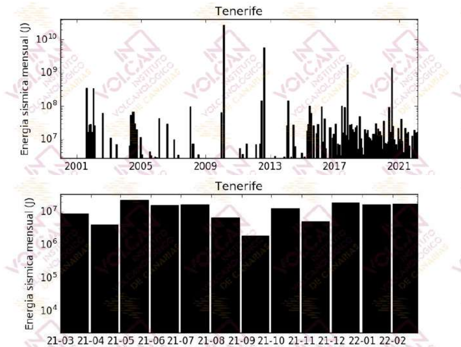
Figura 1.5 – Energía sísmica liberada por los terremotos localizados en el área de Tenerife. El histograma superior corresponde al periodo enero 2001 – febrero 2022, mientras que el inferior muestra el periodo marzo 2021 – febrero 2022. [La fuente de los datos sísmicos anteriores al 21/11/2016 es el Instituto Geográfico Nacional].
