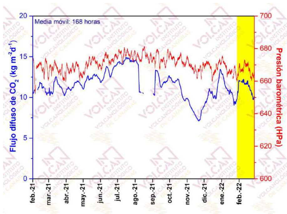
Figura 4.2 - Monitorización de la media móvil semanal del registro en modo continuo del flujo de \text{CO}_2 (azul) y la presión barométrica (rojo) de la estación geoquímica TFG12 (Mirador de la Fortaleza del Teide, Tenerife). Los datos de febrero de 2022 se encuentran indicados por el área amarilla.
