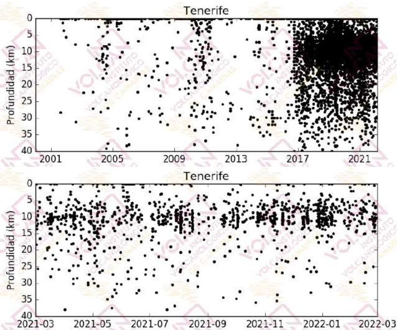
Figura 1.3 - Profundidades de los hipocentros localizados en el área de Tenerife. El gráfico superior corresponde al periodo enero 2001 - febrero 2022, mientras que el inferior muestra el periodo marzo 2021 – febrero 2022. [La fuente de los datos sísmicos anteriores al 21/11/2016 es el Instituto Geográfico Nacional, IGN].
