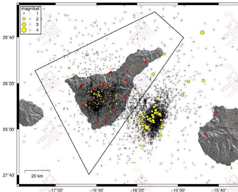
Figura 1.1 - Hipocentros de los terremotos (círculos amarillos) localizados por las estaciones de la Red Sísmica Canaria (triángulos rojos) en febrero de 2022. Las cruces muestran los hipocentros localizados en los últimos 12 meses. El polígono negro corresponde al área de Tenerife considerada en las estadísticas sismológicas de los gráficos siguientes.
