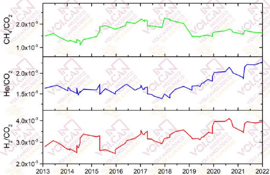
Figura 4.8 - Variaciones temporales de las relaciones molares CO 2 /CH 4 , He/CO 2 y H 2 /CO 2 en las fumarolas del Teide (TEF1) desde 2013. Las curvas representan una media móvil sobre 5 valores de muestreo.
