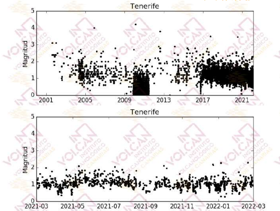
Figura 1.4 - Magnitudes de los terremotos localizados en el área de Tenerife. El gráfico superior corresponde al periodo enero 2001 – febrero 2022, mientras que el inferior muestra el periodo marzo 2021 – febrero 2022. [La fuente de los datos sísmicos anteriores al 21/11/2016 es el Instituto Geográfico Nacional, IGN].
