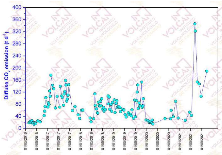
Figura 4.3 – Variaciones temporales de la emisión difusa de dióxido de carbono (CO 2 ) en el cráter del Teide desde el 1 de mayo de 2016 hasta febrero 2022. Los datos de febrero de 2022 se encuentran indicados en azul oscuro.
