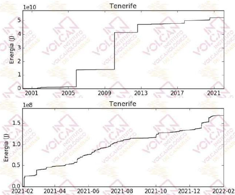
Figura 1.6 - Curva de energía sísmica acumulada por los terremotos localizados en el área de Tenerife. El gráfico superior corresponde al periodo enero 2001 – enero 2022, mientras que el inferior muestra el periodo febrero 2021 – enero 2022. [La fuente de los datos sísmicos anteriores al 21/11/2016 es el Instituto Geográfico Nacional, IGN].
