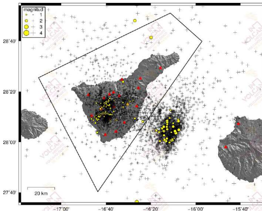
Figura 1.1 - Hipocentros de los terremotos (círculos amarillos) localizados por las estaciones de la Red Sísmica Canaria (triángulos rojos) en enero de 2022. Las cruces muestran los hipocentros localizados en los últimos 12 meses. El polígono negro corresponde al área de Tenerife considerada en las estadísticas sismológicas de los gráficos siguientes.
