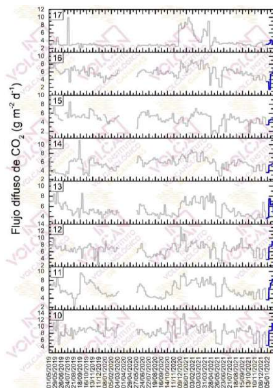
Figura 4.6 – Monitorización semanal del flujo difuso de CO 2 en la Red de Trampas Alcalinas del sistema volcánico Dorsal Norte-Sur de Tenerife desde mayo de 2019. Los datos de enero de 2022 se encuentran indicados en azul oscuro.
