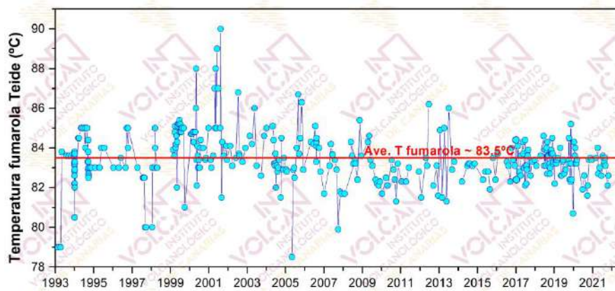
Figura 2.1 – Variaciones temporales de la temperatura registrada en las fumarolas del Teide (TEF1) desde 1993 hasta enero 2022.
