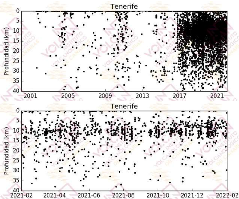
Figura 1.3 - Profundidades de los hipocentros localizados en el área de Tenerife. El gráfico superior corresponde al periodo enero 2001 - enero 2022, mientras que el inferior muestra el periodo febrero 2021 – enero 2022. [La fuente de los datos sísmicos anteriores al 21/11/2016 es el Instituto Geográfico Nacional, IGN].
