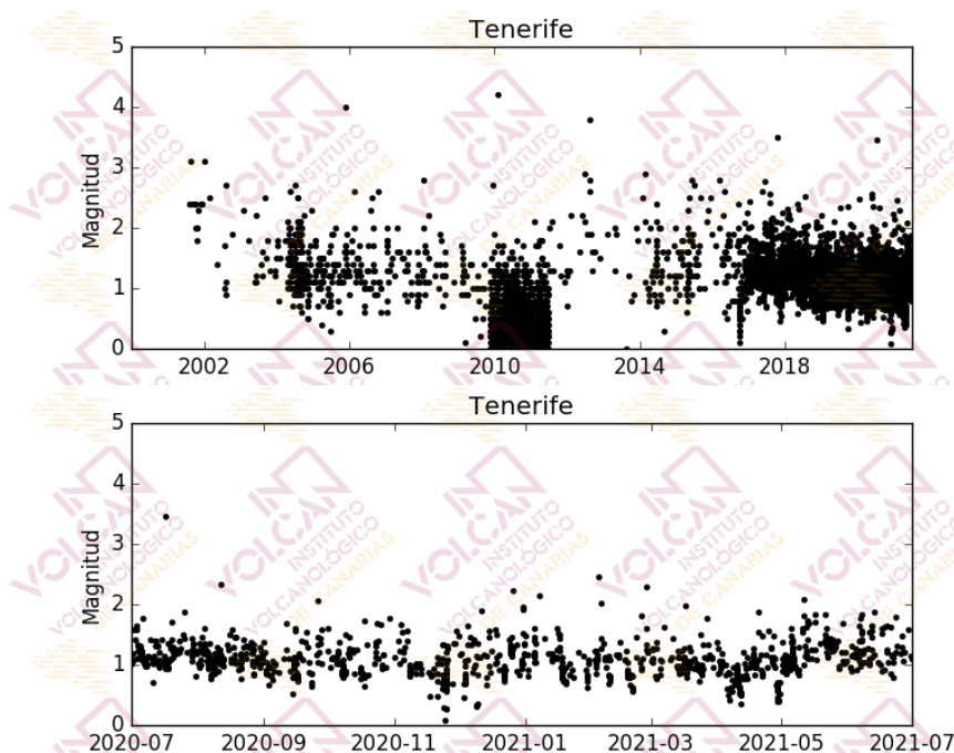
Figura 1.4 - Magnitudes de los terremotos localizados en el área de Tenerife. El gráfico superior corresponde al periodo enero 2000 – junio 2021, mientras que el inferior muestra el periodo julio 2020 – junio 2021. [La fuente de los datos sísmicos anteriores al 21/11/2016 es el Instituto Geográfico Nacional, IGN].
