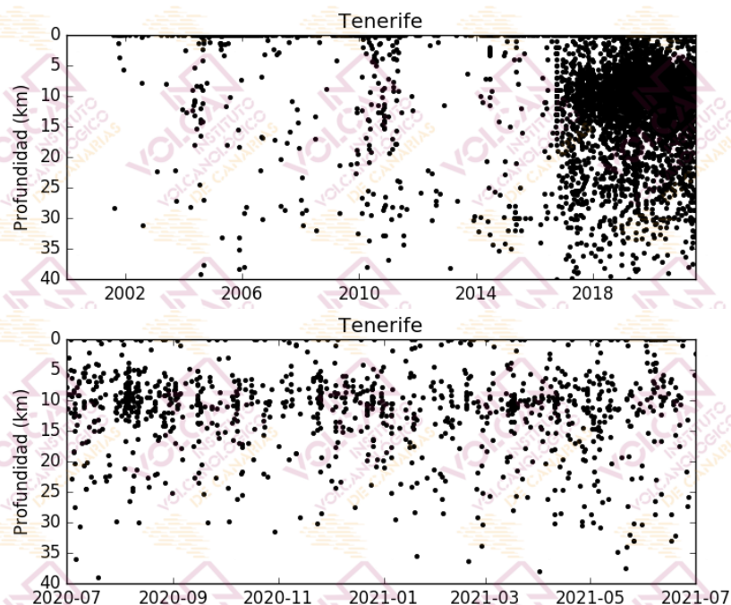
Figura 1.3 - Profundidades de los hipocentros localizados en el área de Tenerife. El gráfico superior corresponde al periodo enero 2000 - junio 2021, mientras que el inferior muestra el periodo julio 2020 – junio 2021. [La fuente de los datos sísmicos anteriores al 21/11/2016 es el Instituto Geográfico Nacional, IGN].
