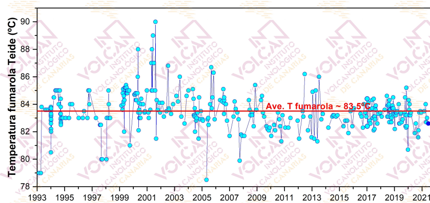
Figura 2.1 – Variaciones temporales de la temperatura registrada en las fumarolas del Teide (TEF1) desde 1993 hasta junio 2021.
