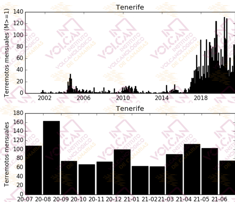
Figura 1.2 - Número de terremotos mensuales en Tenerife. El histograma superior corresponde al periodo enero 2000 – junio 2021 para terremotos con M \geq 1 , mientras que el inferior muestra el periodo julio 2020 – junio 2021 para todas las magnitudes. [La fuente de los datos sísmicos anteriores al 21/11/2016 es el Instituto Geográfico Nacional, IGN].
