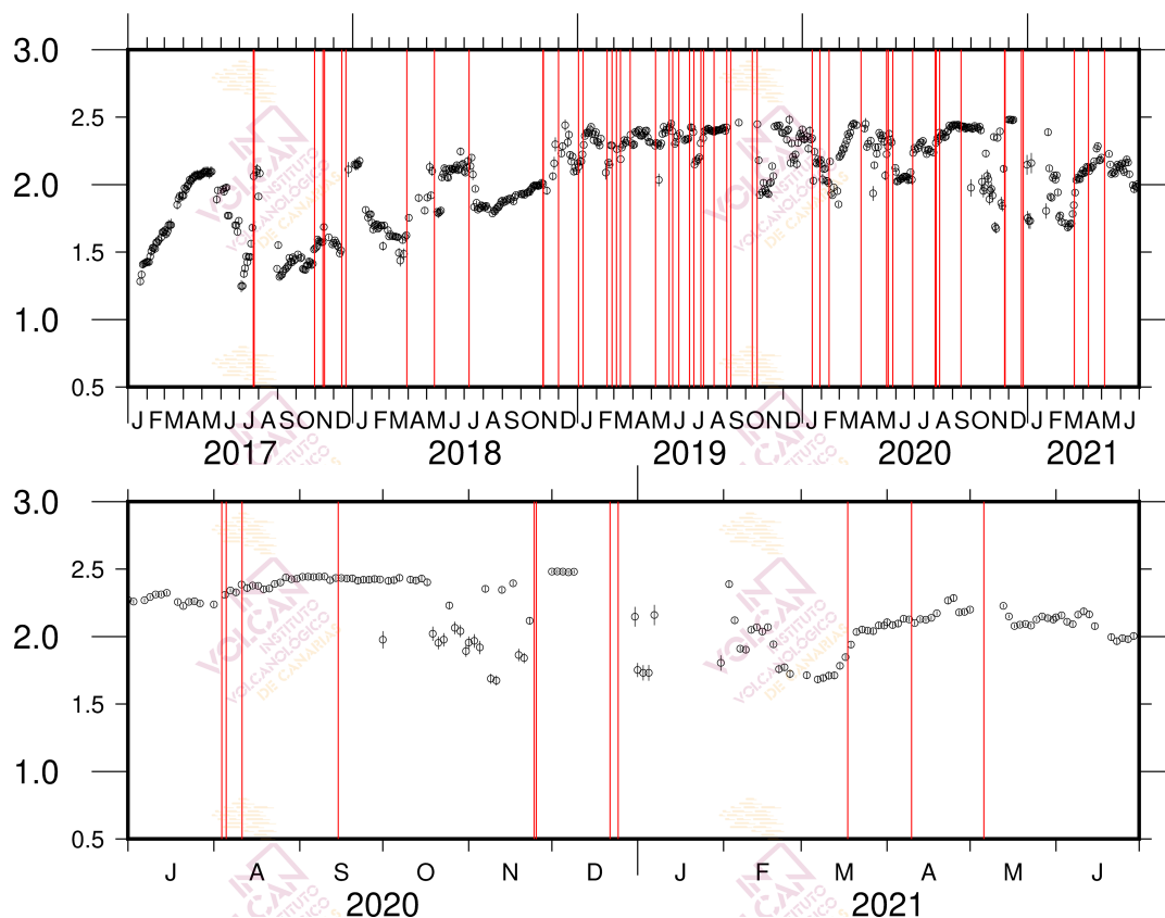
Figura 1.7 - Variaciones del parámetro b de la relación de Gutenberg-Richter. En el gráfico superior durante el periodo enero 2017 – junio 2021. En el gráfico inferior durante el periodo julio 2020 – junio 2021. Las líneas rojas indican la ocurrencia de enjambres sísmicos.
