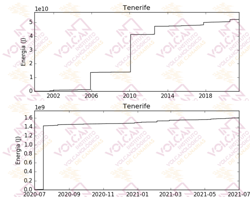
Figura 1.6 - Curva de energía sísmica acumulada por los terremotos localizados en el área de Tenerife. El gráfico superior corresponde al periodo enero 2000 – junio 2021, mientras que el inferior muestra el periodo julio 2020 – junio 2021. [La fuente de los datos sísmicos anteriores al 21/11/2016 es el Instituto Geográfico Nacional, IGN].
