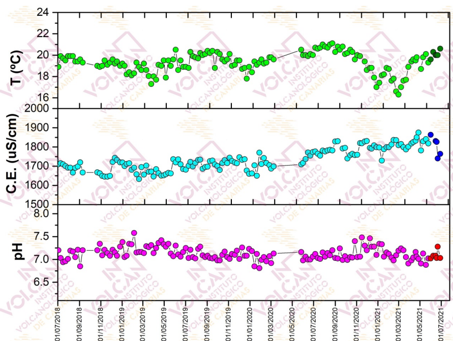
Figura 4.9 - Variaciones temporales de temperatura, conductividad ( \mu S\cdot cm^{-1} ) y pH medidas en el agua subterránea de la estación geoquímica TFG03. Los datos de junio de 2021 se encuentran indicados en diferentes colores.
