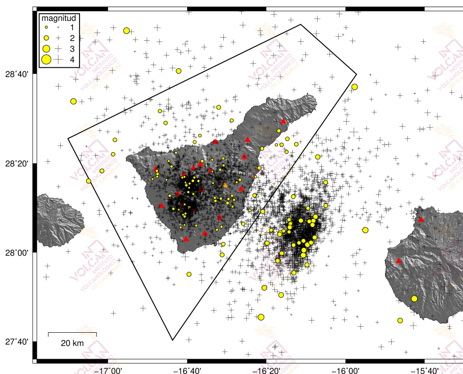
Figura 1.1 - Hipocentros de los terremotos (círculos amarillos) localizados por las estaciones de la Red Sísmica Canaria (triángulos rojos) en junio de 2021. Las cruces muestran los hipocentros localizados en los últimos 12 meses. El polígono negro corresponde al área de Tenerife considerada en las estadísticas sismológicas de los gráficos siguientes.
