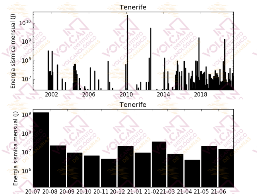
Figura 1.5 – Energía sísmica liberada por los terremotos localizados en el área de Tenerife. El histograma superior corresponde al periodo enero 2000 – junio 2021, mientras que el inferior muestra el periodo julio 2020 – junio 2021. [La fuente de los datos sísmicos anteriores al 21/11/2016 es el Instituto Geográfico Nacional].
