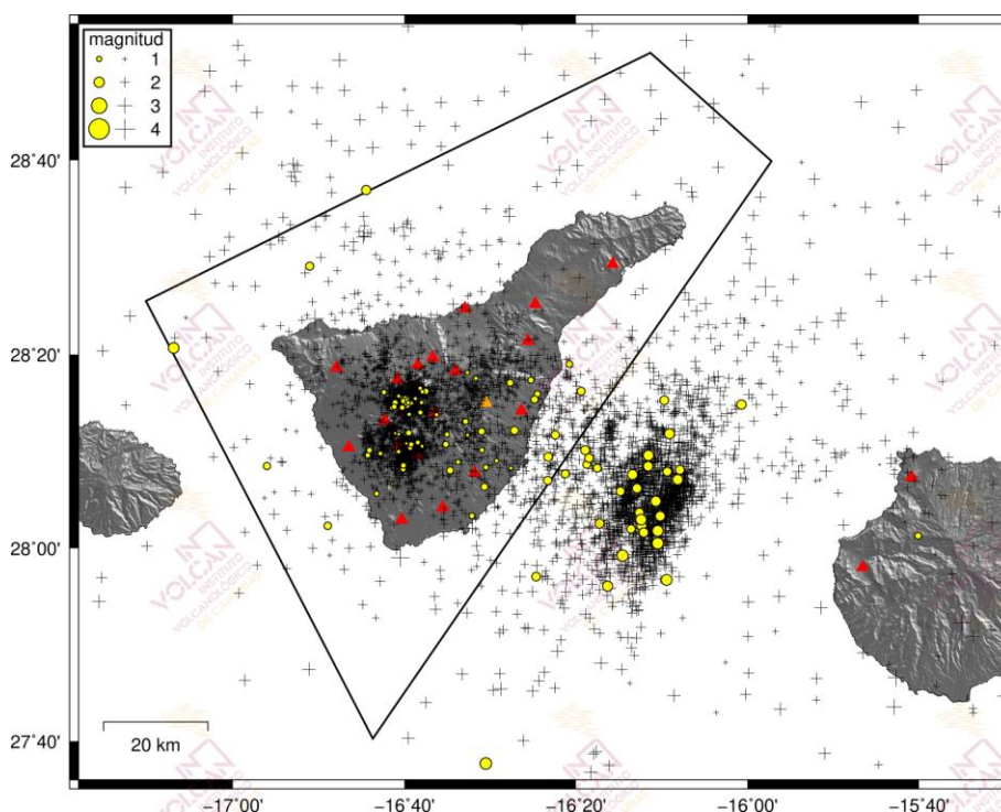
Figura 1.1 - Hipocentros de los terremotos (círculos amarillos) localizados por las estaciones de la Red Sísmica Canaria (triángulos rojos) en septiembre de 2020. Las cruces muestran los hipocentros localizados en los últimos 12 meses. El polígono negro corresponde al área de Tenerife considerada en las estadísticas sismológicas de los gráficos siguientes.
