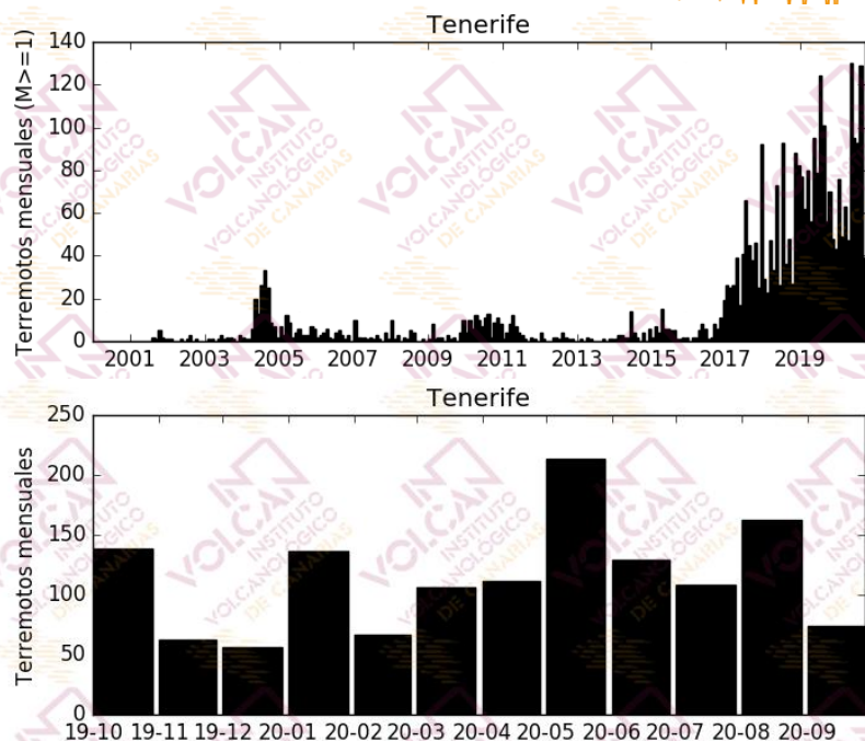
Figura 1.2 - Número de terremotos mensuales en Tenerife. El histograma superior corresponde al periodo enero 2000 – septiembre 2020 para terremotos con M \geq 1 , mientras que el inferior muestra el periodo octubre 2019 – septiembre 2020 para todas las magnitudes. [La fuente de los datos sísmicos anteriores al 21/11/2016 es el Instituto Geográfico Nacional, IGN].
