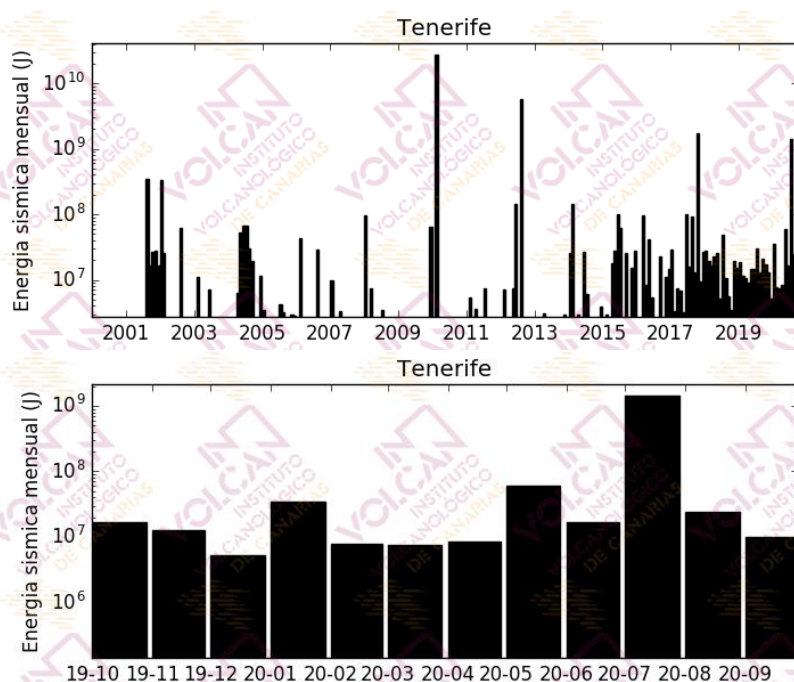
Figura 1.5 – Energía sísmica liberada por los terremotos localizados en el área de Tenerife. El histograma superior corresponde al periodo enero 2000 – septiembre 2020, mientras que el inferior muestra el periodo octubre 2019 – septiembre 2020. [La fuente de los datos sísmicos anteriores al 21/11/2016 es el Instituto Geográfico Nacional].
