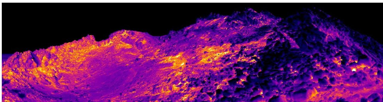
Figura 2.4. Imagen térmica del cráter del Teide obtenida con cámara la térmica FLIR T660.
