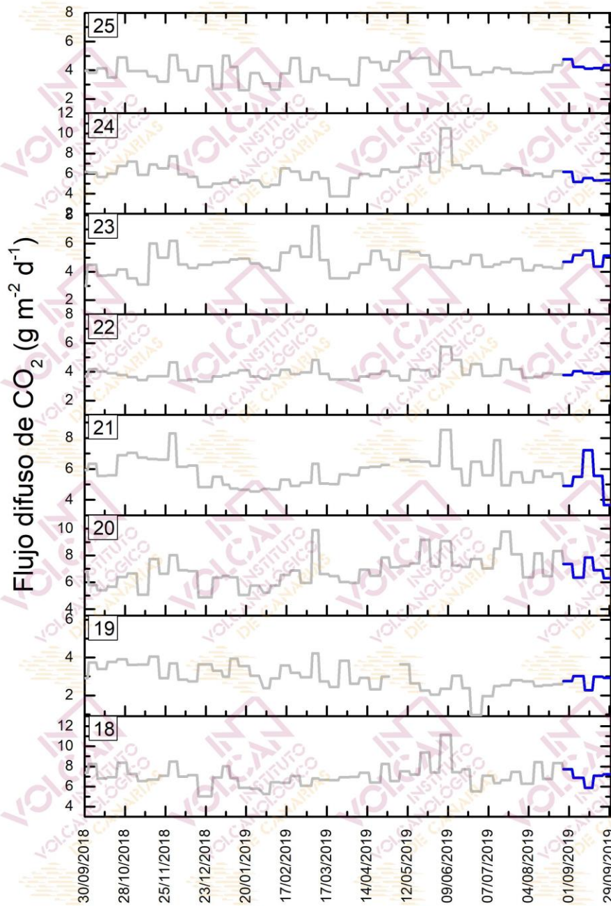
Figura 4.7 – Monitorización semanal del flujo difuso de \text{CO}_2 en la Red de Trampas Alcalinas de la Caldera de Las Cañadas durante los últimos 12 meses. Los datos de septiembre de 2019 se encuentran marcados en azul oscuro.
