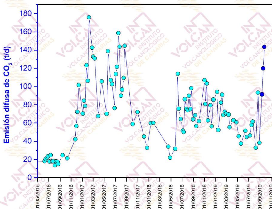
Figura 4.3 – Variaciones temporales de la emisión difusa de dióxido de carbono ( \text{CO}_2 ) en el cráter del Teide desde el 1 de junio de 2016. Los datos de septiembre de 2019 se encuentran marcados en azul oscuro.
