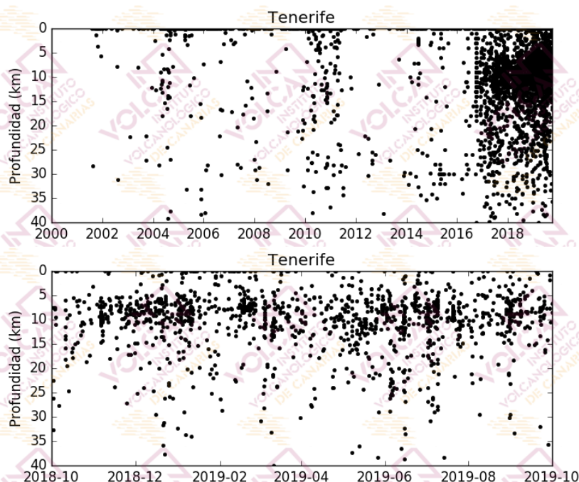
Figura 1.3 - Profundidades de los hipocentros localizados en el área de Tenerife. El gráfico superior corresponde al periodo enero 2000 - septiembre 2019, mientras que el inferior muestra el periodo octubre 2018 - septiembre 2019. [La fuente de los datos sísmicos anteriores al 21/11/2016 es el Instituto Geográfico Nacional, IGN].
