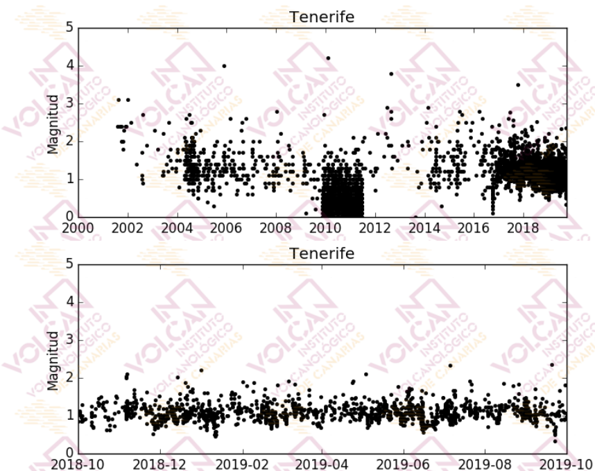
Figura 1.4 - Magnitudes de los terremotos localizados en el área de Tenerife. El gráfico superior corresponde al periodo enero 2000 - septiembre 2019, mientras que el inferior muestra el periodo octubre 2018 - septiembre 2019. [La fuente de los datos sísmicos anteriores al 21/11/2016 es el Instituto Geográfico Nacional, IGN].
