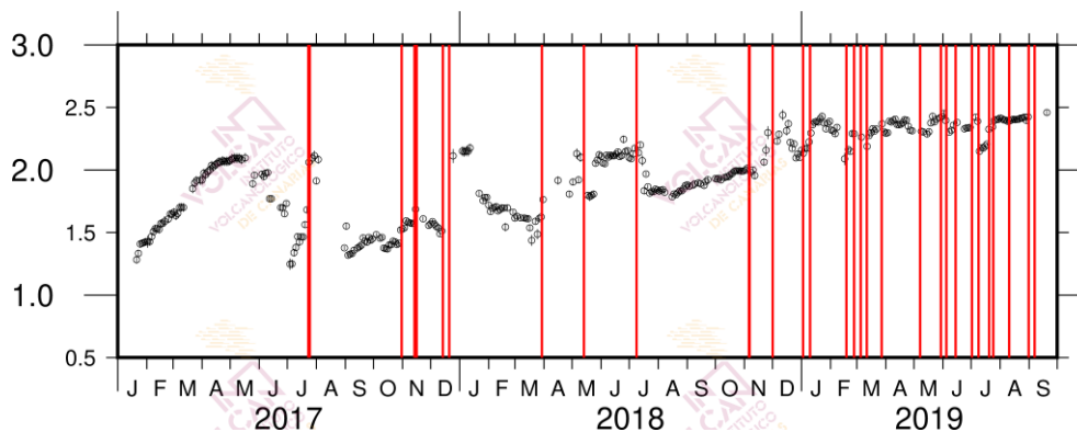
Figura 1.7 - Variaciones del parámetro b de la relación de Gutenberg-Richter durante el período enero 2017 - septiembre 2019. Las líneas rojas indican la ocurrencia de enjambres sísmicos.
