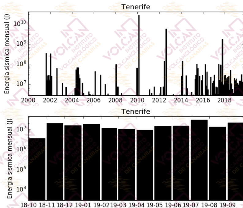
Figura 1.5 – Energía sísmica liberada por los terremotos localizados en el área de Tenerife. El histograma superior corresponde al periodo enero 2000 - septiembre 2019, mientras que el inferior muestra el periodo octubre 2018 - septiembre 2019. [La fuente de los datos sísmicos anteriores al 21/11/2016 es el Instituto Geográfico Nacional].
