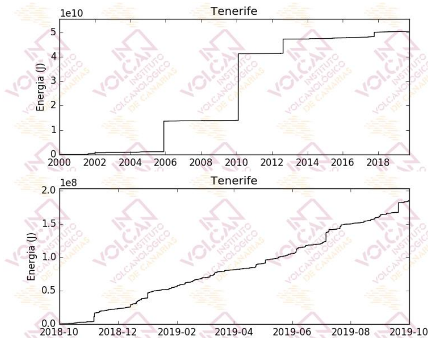
Figura 1.6 - Curva de energía sísmica acumulada por los terremotos localizados en el área de Tenerife. El gráfico superior corresponde al periodo enero 2000 - septiembre 2019, mientras que el inferior muestra el periodo octubre 2018 - septiembre 2019. [La fuente de los datos sísmicos anteriores al 21/11/2016 es el Instituto Geográfico Nacional, IGN].
