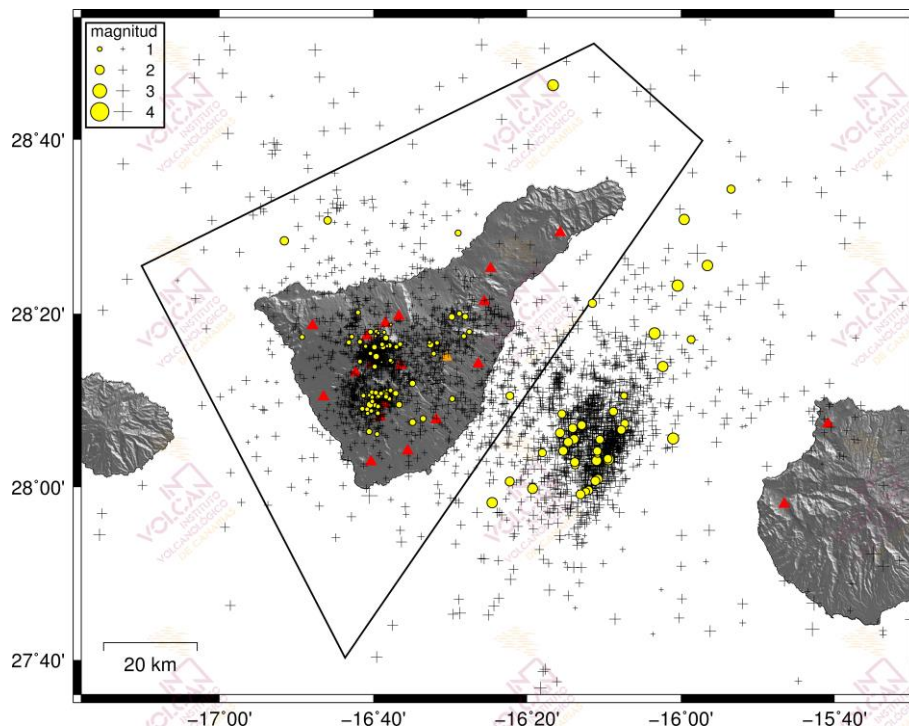
Figura 1.1 - Hipocentros de los terremotos (círculos amarillos) localizados por las estaciones de la Red Sísmica Canaria (triángulos rojos) en septiembre de 2019. Las cruces muestran los hipocentros localizados en los últimos 12 meses. El polígono negro corresponde al área de Tenerife considerada en las estadísticas sísmológicas de los gráficos siguientes.
