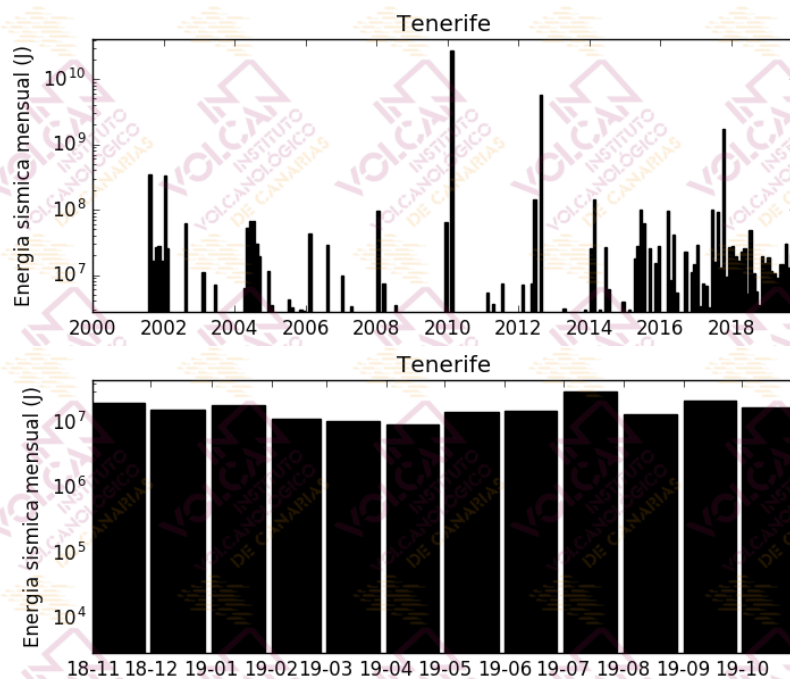
Figura 1.5 - Energía sísmica liberada por los terremotos localizados en el área de Tenerife. El histograma superior corresponde al periodo enero 2000 - octubre 2019, mientras que el inferior muestra el periodo noviembre 2018 - octubre 2019. [La fuente de los datos sísmicos anteriores al 21/11/2016 es el Instituto Geográfico Nacional].
