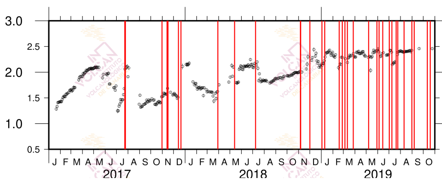
Figura 1.7 - Variaciones del parámetro b de la relación de Gutenberg-Richter durante el periodo enero 2017 - octubre 2019. Las líneas rojas indican la ocurrencia de enjambres sísmicos.
