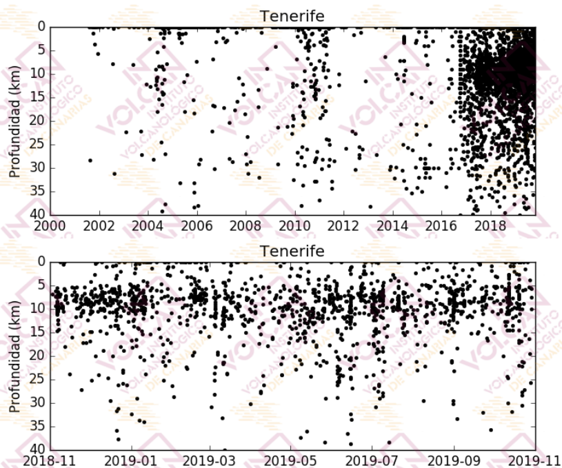
Figura 1.3 - Profundidades de los hipocentros localizados en el área de Tenerife. El gráfico superior corresponde al periodo enero 2000 - octubre 2019, mientras que el inferior muestra el periodo noviembre 2018 - octubre 2019. [La fuente de los datos sísmicos anteriores al 21/11/2016 es el Instituto Geográfico Nacional, IGN].
