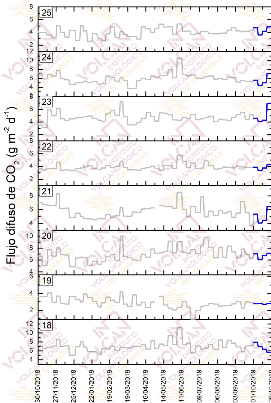
Figura 4.7 – Monitorización semanal del flujo difuso de \text{CO}_2 en la Red de Trampas Alcalinas de la Caldera de Las Cañadas durante los últimos 12 meses. Los datos de octubre de 2019 se encuentran marcados en azul oscuro.
