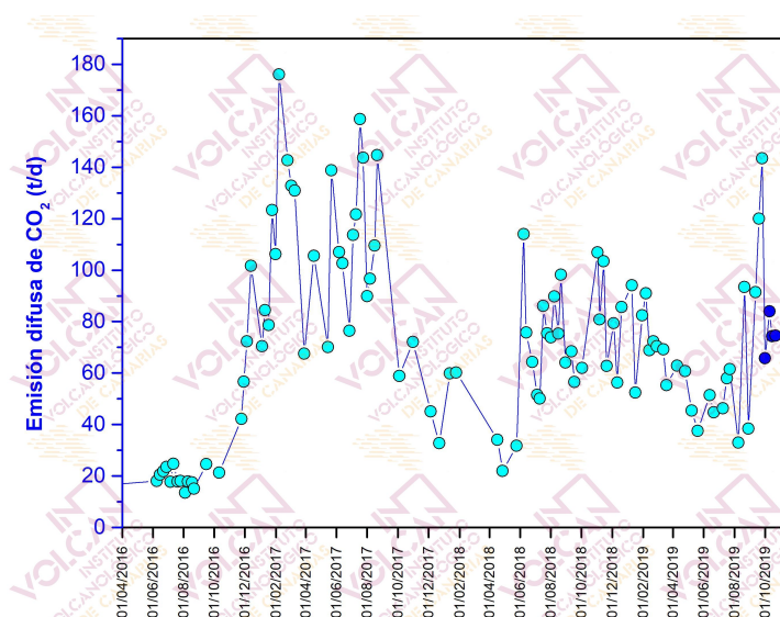
Figura 4.3 – Variaciones temporales de la emisión difusa de dióxido de carbono ( \text{CO}_2 ) en el cráter del Teide desde el 1 de junio de 2016. Los datos de octubre de 2019 se encuentran marcados en azul oscuro.
