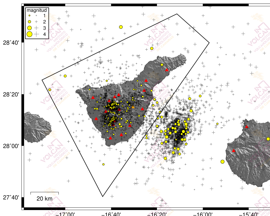
Figura 1.1 - Hipocentros de los terremotos (círculos amarillos) localizados por las estaciones de la Red Sísmica Canaria (triángulos rojos) en octubre de 2019. Las cruces muestran los hipocentros localizados en los últimos 12 meses. El polígono negro corresponde al área de Tenerife considerada en las estadísticas sísmológicas de los gráficos siguientes.
