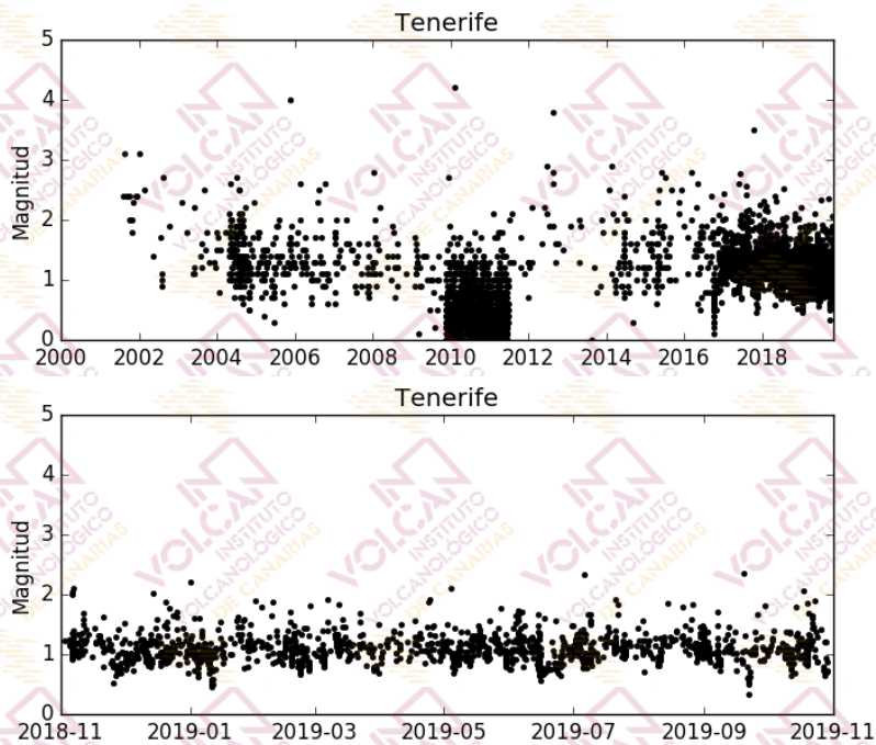
Figura 1.4 - Magnitudes de los terremotos localizados en el área de Tenerife. El gráfico superior corresponde al periodo enero 2000 - octubre 2019, mientras que el inferior muestra el periodo noviembre 2018 - octubre 2019. [La fuente de los datos sísmicos anteriores al 21/11/2016 es el Instituto Geográfico Nacional, IGN].
