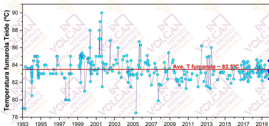
Figura 2.1 – Variaciones temporales de la temperatura registrada en las fumarolas del Teide (TEF1) desde 1993. Los datos de octubre de 2019 se encuentran marcados en azul oscuro.
