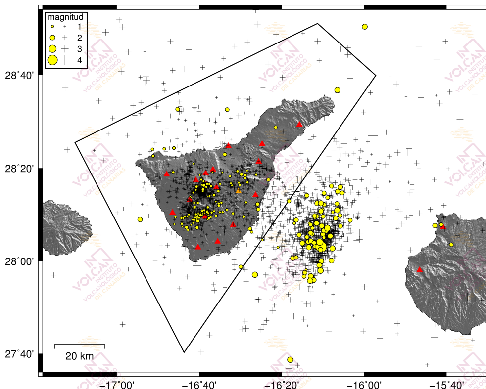
Figura 1.1 - Hipocentros de los terremotos (círculos amarillos) localizados por las estaciones de la Red Sísmica Canaria (triángulos rojos) en enero de 2019. Las cruces muestran los hipocentros localizados en los últimos 12 meses. El polígono negro corresponde al área de Tenerife considerada en las estadísticas sísmológicas de los gráficos siguientes.
