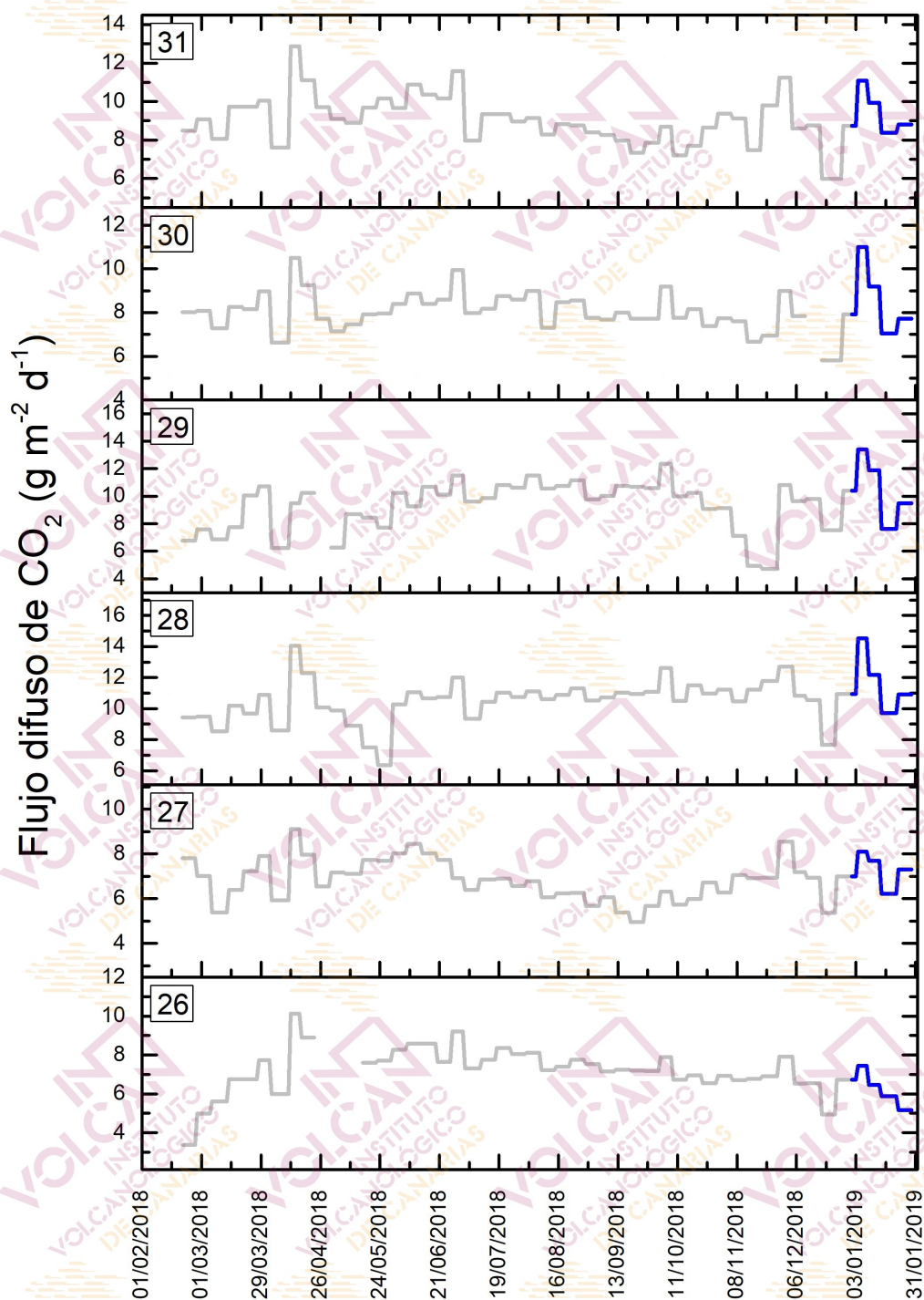
Figura 4.5 – Monitorización semanal del flujo difuso de CO 2 en la Red de Trampas Alcalinas del sistema volcánico Dorsal Noreste de Tenerife durante los últimos 12 meses. Los datos de enero de 2019 se encuentran marcados en azul oscuro.
