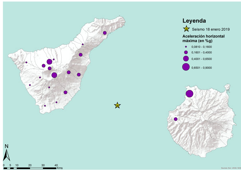
Figura 1.8 - Aceleraciones máximas horizontales (PGA) por el terremoto del 18 de enero con M=4,4 .
