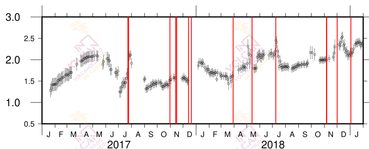
Figura 1.7 - Variaciones del parámetro b de la relación de Gutenberg-Richter desde enero 2017 hasta enero 2019. Las líneas rojas indican la ocurrencia de enjambres sísmicos.
