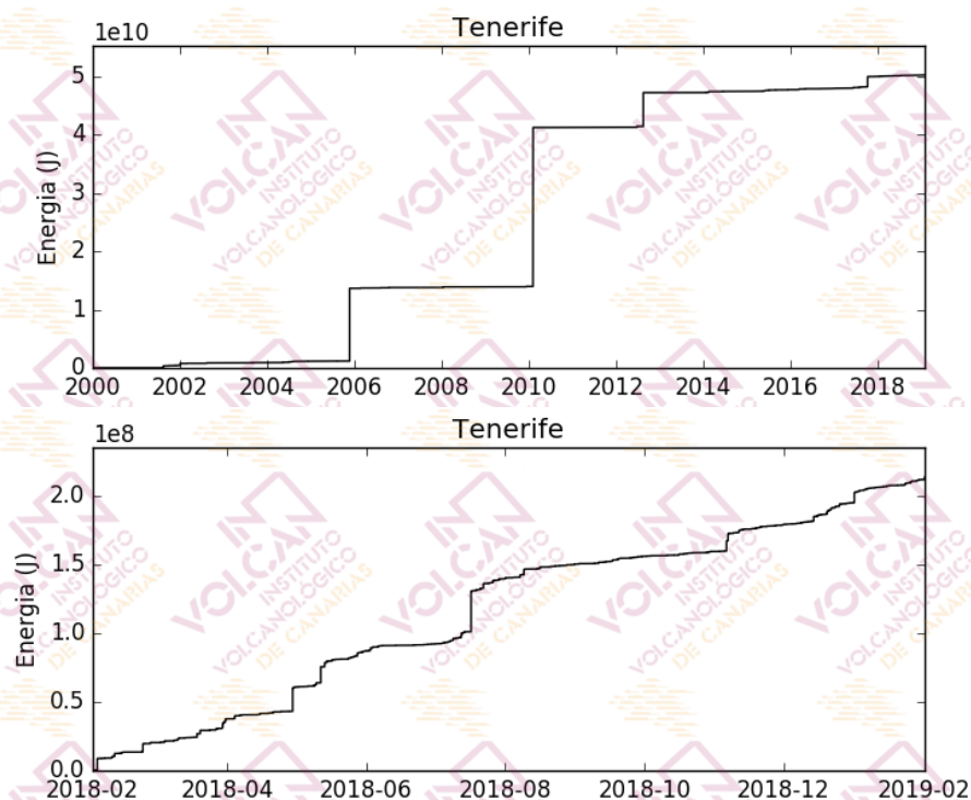
Figura 1.6 - Curva de energía sísmica acumulada por los terremotos localizados en el área de Tenerife. El gráfico superior corresponde al periodo enero 2000- enero 2019, mientras que el inferior muestra el periodo febrero 2018-enero 2019. [La fuente de los datos sísmicos anteriores al 21/11/2016 es el Instituto Geográfico Nacional, IGN].
