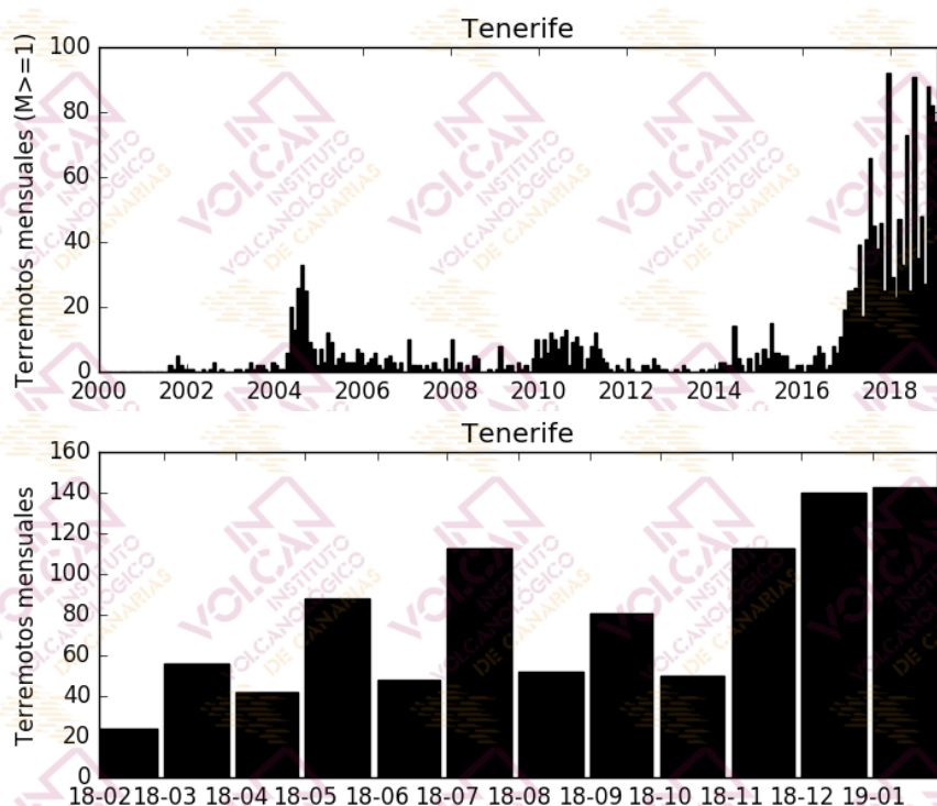
Figura 1.2 - Número de terremotos mensuales en Tenerife. El histograma superior corresponde al periodo enero 2000-enero 2019 para terremotos con M \geq 1 , mientras que el inferior muestra el periodo febrero 2018-enero 2019 para todas las magnitudes. [La fuente de los datos sísmicos anteriores al 21/11/2016 es el Instituto Geográfico Nacional, IGN].
