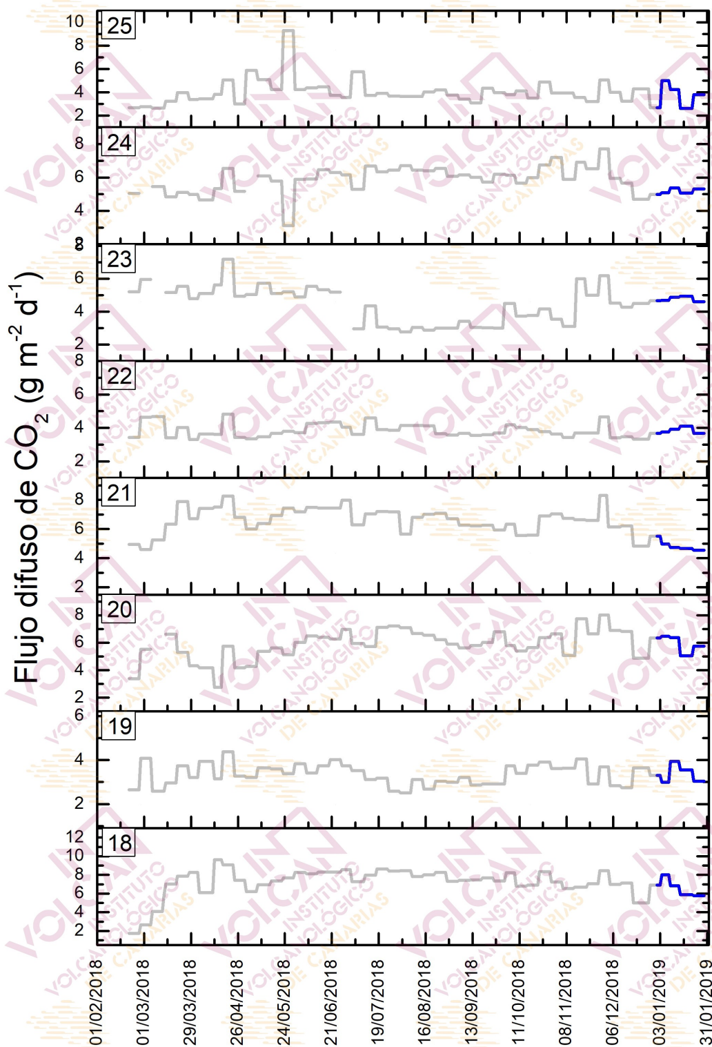
Figura 4.7 – Monitorización semanal del flujo difuso de CO 2 en la Red de Trampas Alcalinas de la Caldera de Las Cañadas durante los últimos 12 meses. Los datos de enero de 2019 se encuentran marcados en azul oscuro.
