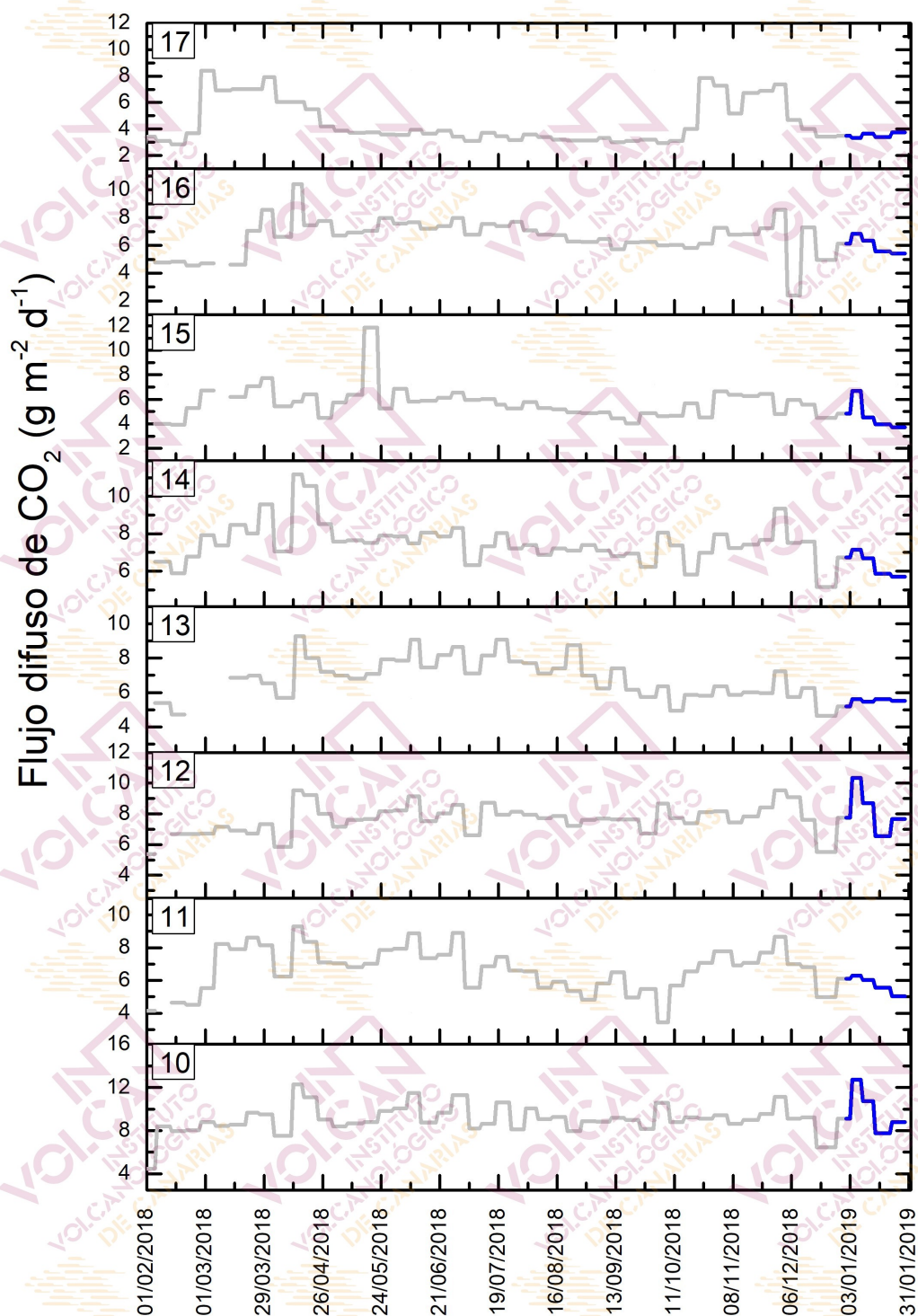
Figura 4.6 – Monitorización semanal del flujo difuso de \text{CO}_2 en la Red de Trampas Alcalinas del sistema volcánico Dorsal Norte-Sur de Tenerife durante los últimos 12 meses. Los datos de enero de 2019 se encuentran marcados en azul oscuro.
