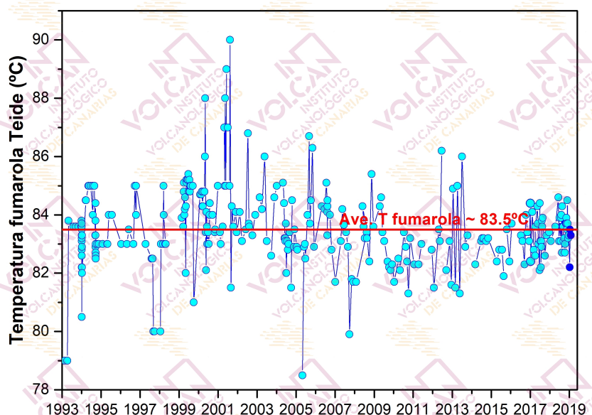
Figura 2.1 – Variaciones temporales de la temperatura registrada en las fumarolas del Teide (TEF1) desde 1993. Los datos de enero de 2019 se encuentran marcados en azul oscuro.
