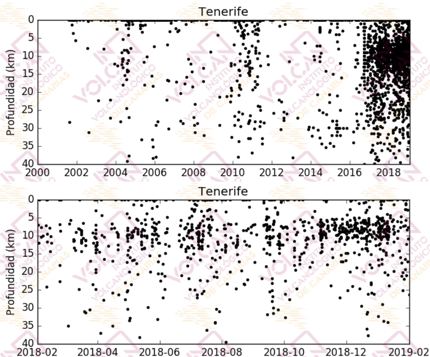
Figura 1.3 - Profundidades de los hipocentros localizados en el área de Tenerife. El gráfico superior corresponde al periodo enero 2000-enero 2019, mientras que el inferior muestra el periodo febrero 2018-enero 2019. [La fuente de los datos sísmicos anteriores al 21/11/2016 es el Instituto Geográfico Nacional, IGN].
