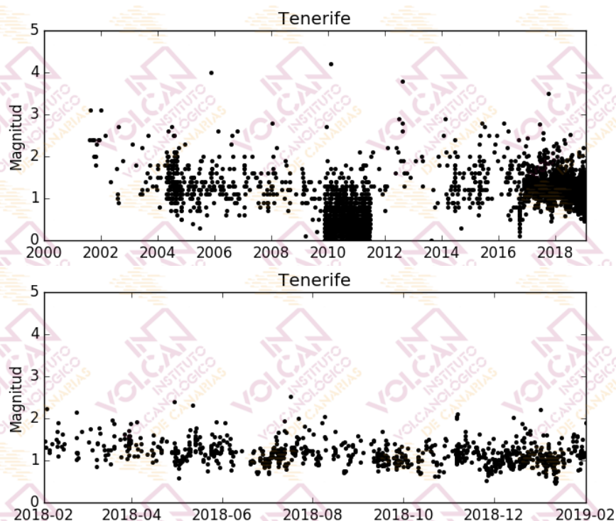
Figura 1.4 - Magnitudes de los terremotos localizados en el área de Tenerife. El gráfico superior corresponde al periodo enero 2000- enero 2019, mientras que el inferior muestra el periodo febrero 2018-enero 2019. [La fuente de los datos sísmicos anteriores al 21/11/2016 es el Instituto Geográfico Nacional, IGN].
