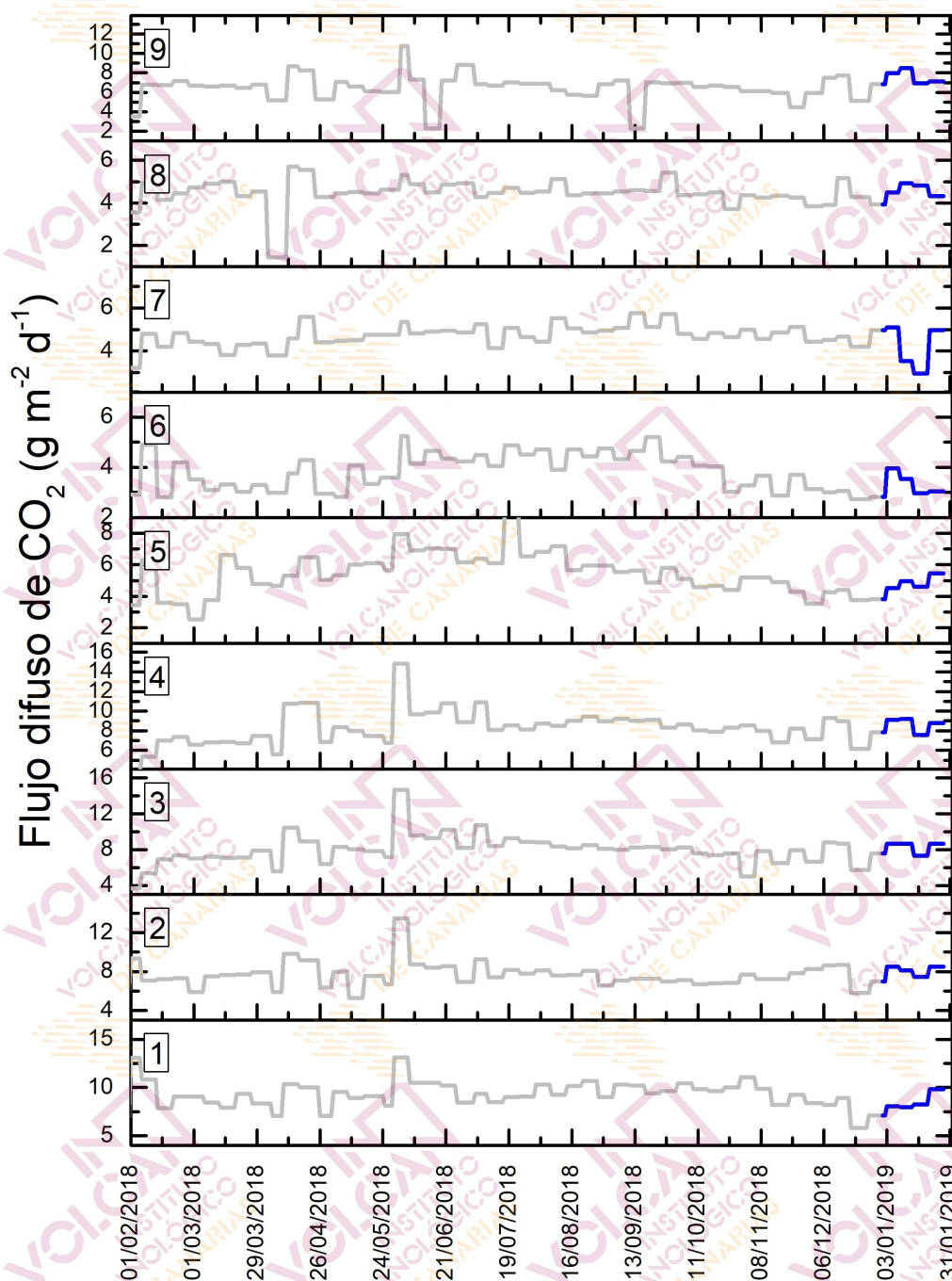
Figura 4.4 – Monitorización semanal del flujo difuso de CO 2 en la Red de Trampas Alcalinas del sistema volcánico Dorsal Noroeste de Tenerife durante los últimos 12 meses. Los datos de enero de 2019 se encuentran marcados en azul oscuro.
