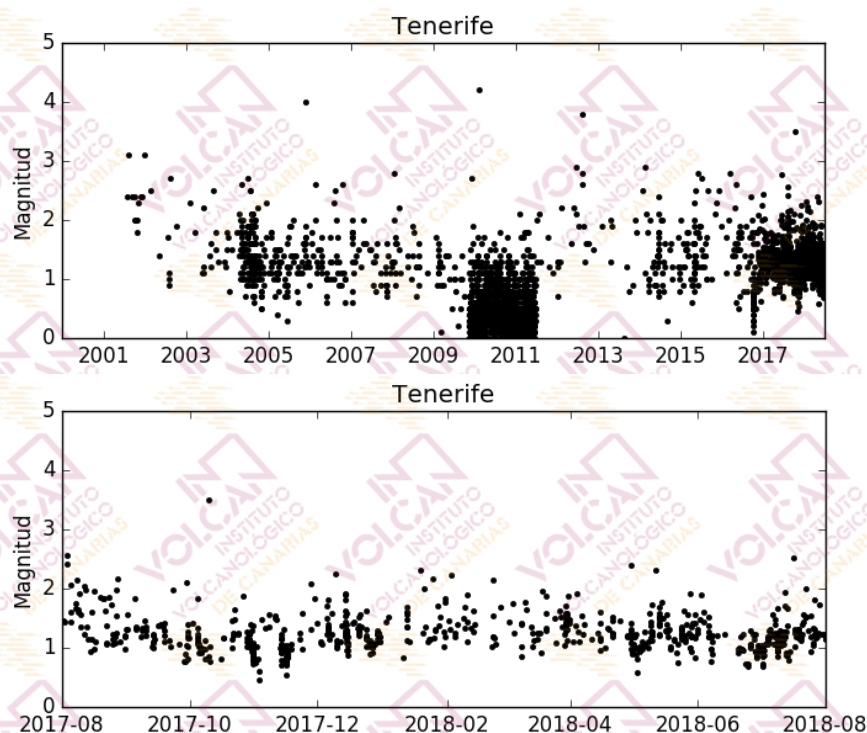
Figura 1.4 - Magnitudes de los terremotos localizados en el área de Tenerife. El gráfico superior corresponde al periodo enero 2000-julio 2018, mientras que el inferior muestra el periodo agosto 2017-julio 2018. [La fuente de los datos sísmicos anteriores al 21/11/2016 es el Instituto Geográfico Nacional, IGN].
