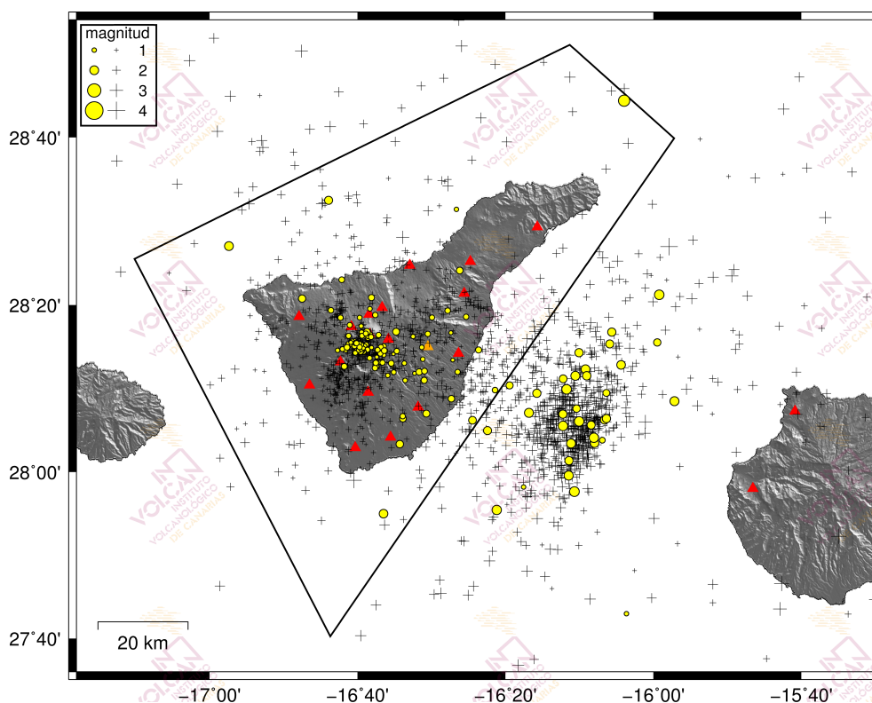
Figura 1.1 - Hipocentros de los terremotos (círculos amarillos) localizados por las estaciones de la Red Sísmica Canaria (triángulos rojos) en julio de 2018. Las cruces muestran los hipocentros localizados en los últimos 12 meses. El polígono negro corresponde al área de Tenerife considerada en las estadísticas sísmológicas de los gráficos siguientes.
