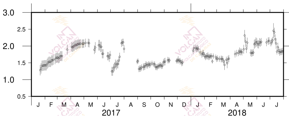
Figura 1.7 - Variaciones del parámetro b de la relación de Gutenberg-Richter desde enero 2017 hasta julio 2018.
