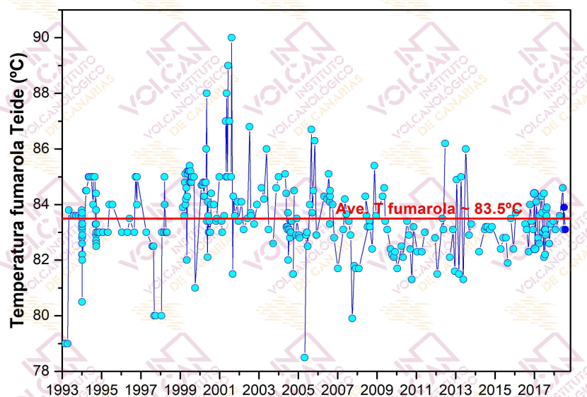
Figura 2.1 – Variaciones temporales de la temperatura registrada en la fumarola del Teide (TEF1) desde 1993. Los datos de julio de 2018 se encuentran marcados en azul oscuro.
