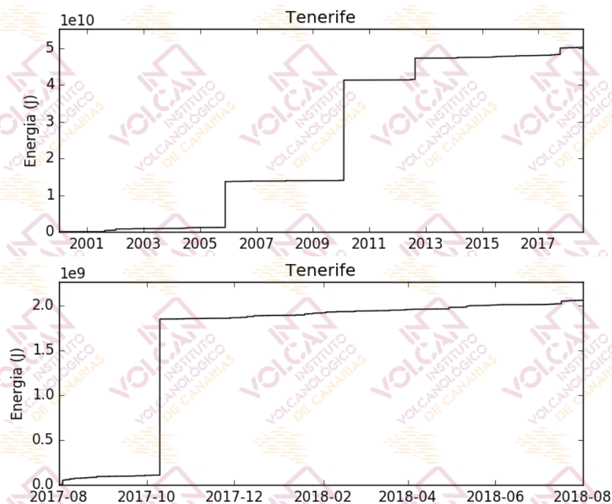
Figura 1.6 - Curva de energía sísmica acumulada por los terremotos localizados en el área de Tenerife. El gráfico superior corresponde al periodo enero 2000-julio 2018, mientras que el inferior muestra el periodo agosto 2017-julio 2018. [La fuente de los datos anteriores al 21/11/2016 es el Instituto Geográfico Nacional, IGN].
