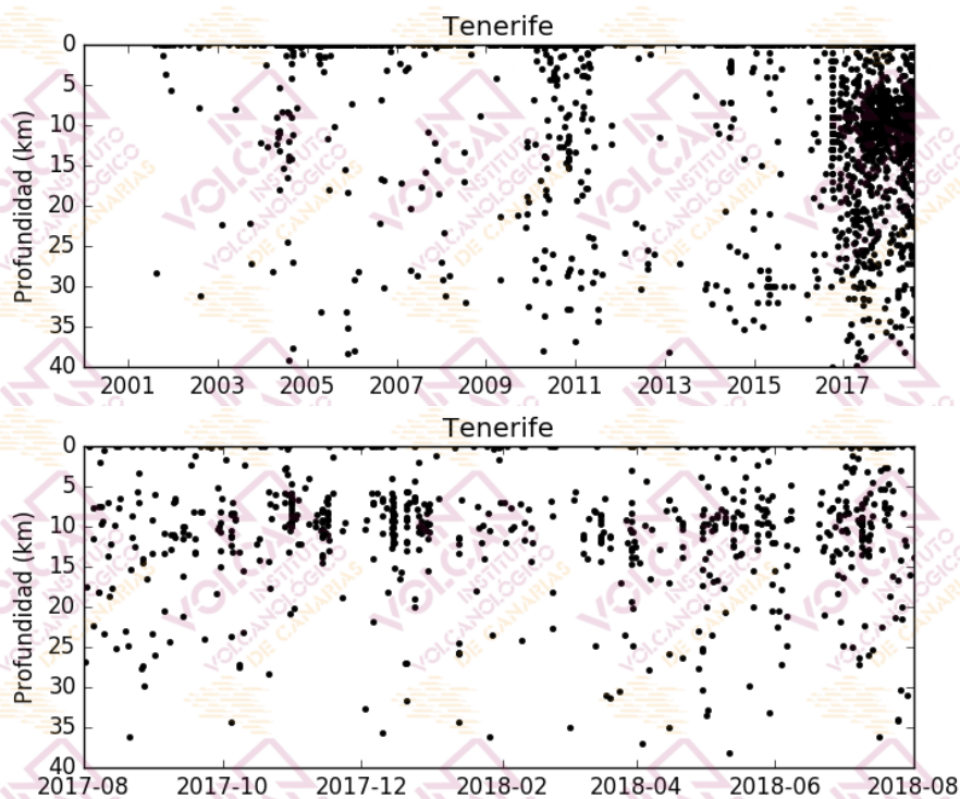
Figura 1.3 - Profundidades de los hipocentros localizados en el área de Tenerife. El gráfico superior corresponde al periodo enero 2000-julio 2018, mientras que el inferior muestra el periodo julio 2017-julio 2018. [La fuente de los datos sísmicos anteriores al 21/11/2016 es el Instituto Geográfico Nacional, IGN].
