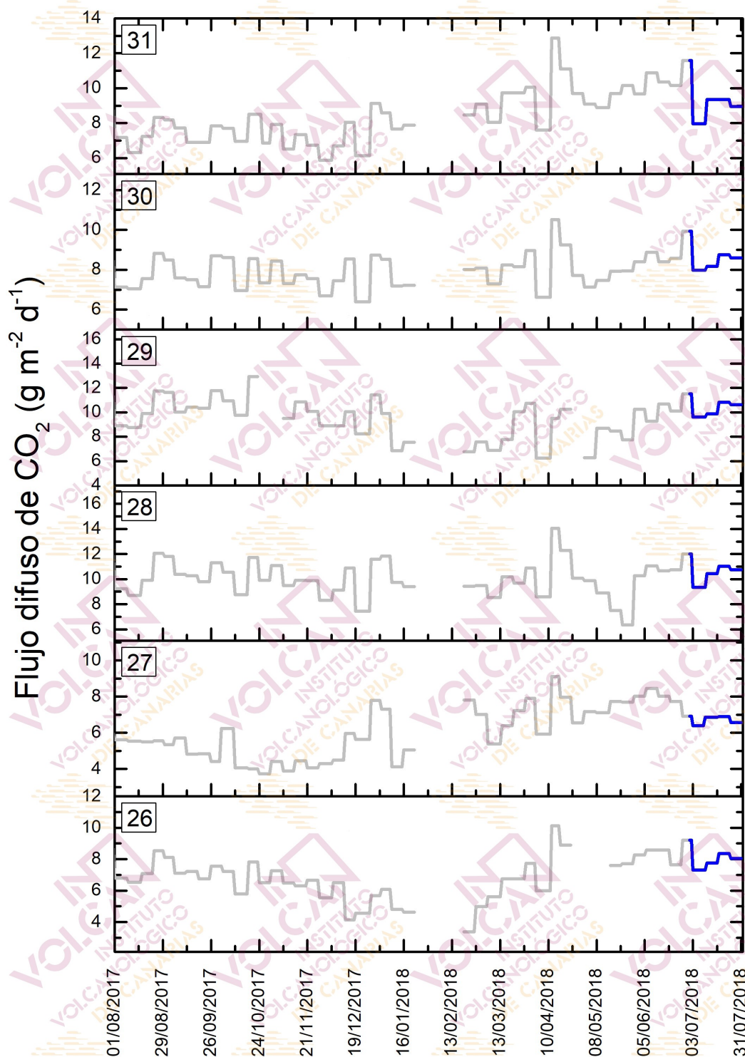
Figura 4.5 – Monitorización semanal del flujo difuso de CO 2 en la Red de Trampas Alcalinas del sistema volcánico Dorsal Noreste de Tenerife durante los últimos 12 meses. Los datos de julio de 2018 se encuentran marcados en azul oscuro.
