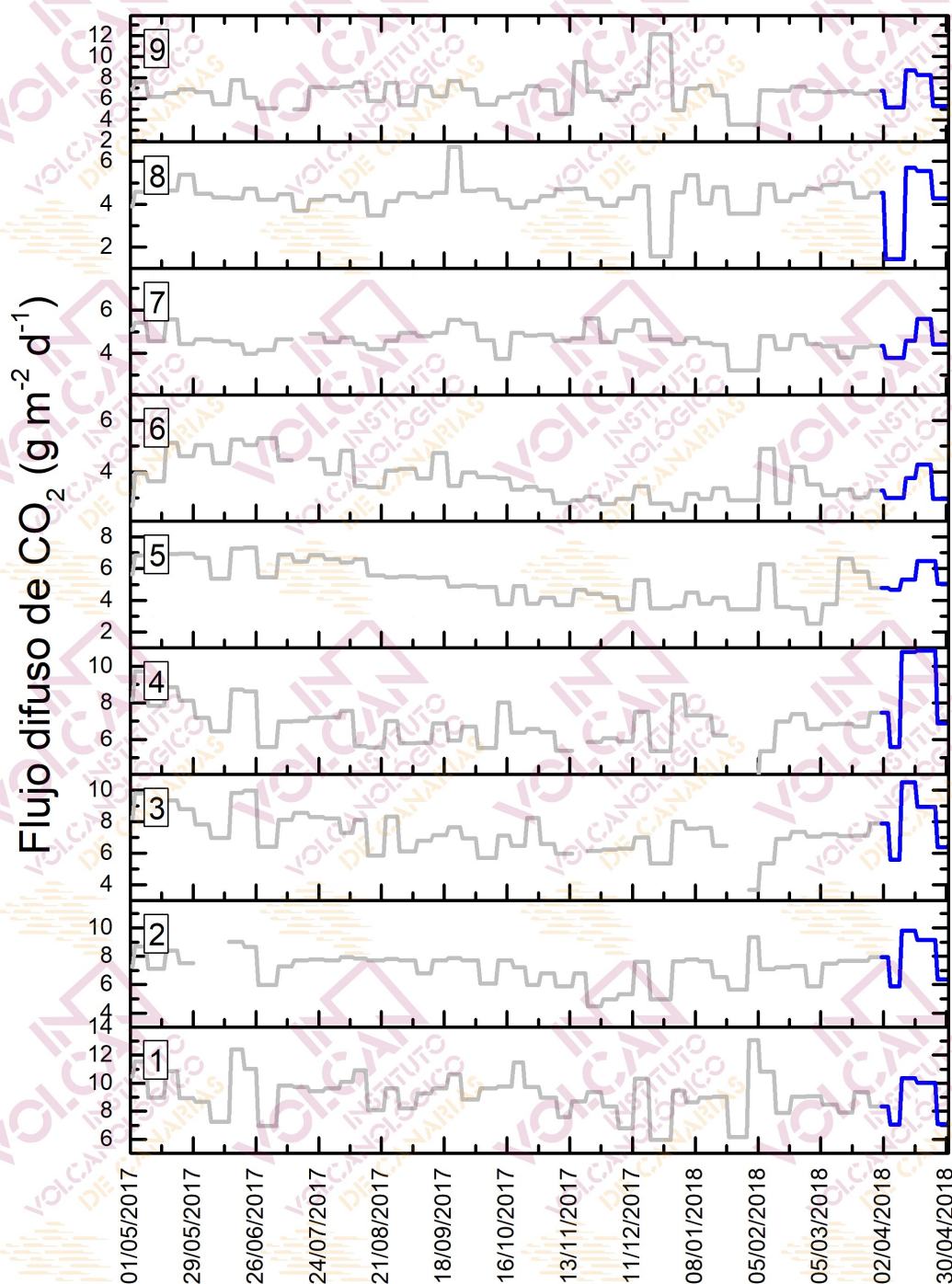
Figura 4.4 – Monitorización semanal del flujo difuso de CO 2 en la Red de Trampas Alcalinas del sistema volcánico Dorsal Noroeste de Tenerife durante los últimos 12 meses. Los datos de abril de 2018 se encuentran marcados en azul oscuro.
