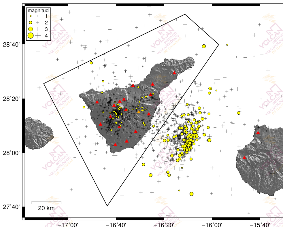
Figura 1.1 - Hipocentros de los terremotos (círculos amarillos) localizados por las estaciones de la Red Sísmica Canaria (triángulos rojos) en abril de 2018. Las cruces muestran los hipocentros localizados en los últimos 12 meses. El polígono negro corresponde al área de Tenerife considerada en las estadísticas sismológicas de los gráficos siguientes.
