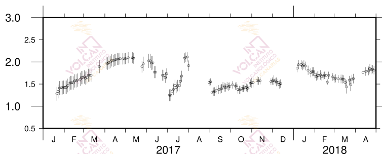
Figura 1.7 - Variaciones del parámetro b de la relación de Gutenberg-Richter desde enero 2017 hasta abril 2018.
