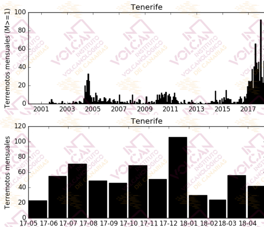
Figura 1.2 - Número de terremotos mensuales en Tenerife. El histograma superior corresponde al periodo enero 2000-abril 2018 para terremotos con M \geq 1 , mientras que el inferior muestra el periodo mayo 2017-abril 2018 para todas las magnitudes. [La fuente de los datos sísmicos anteriores al 21/11/2016 es el Instituto Geográfico Nacional, IGN].
