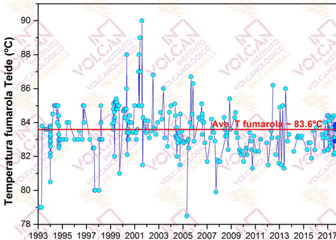
Figura 2.1 – Variaciones temporales de la temperatura registrada en la fumarola del Teide (TEF1) desde 1993. Los datos de agosto de 2017 se marcan en azul oscuro.
