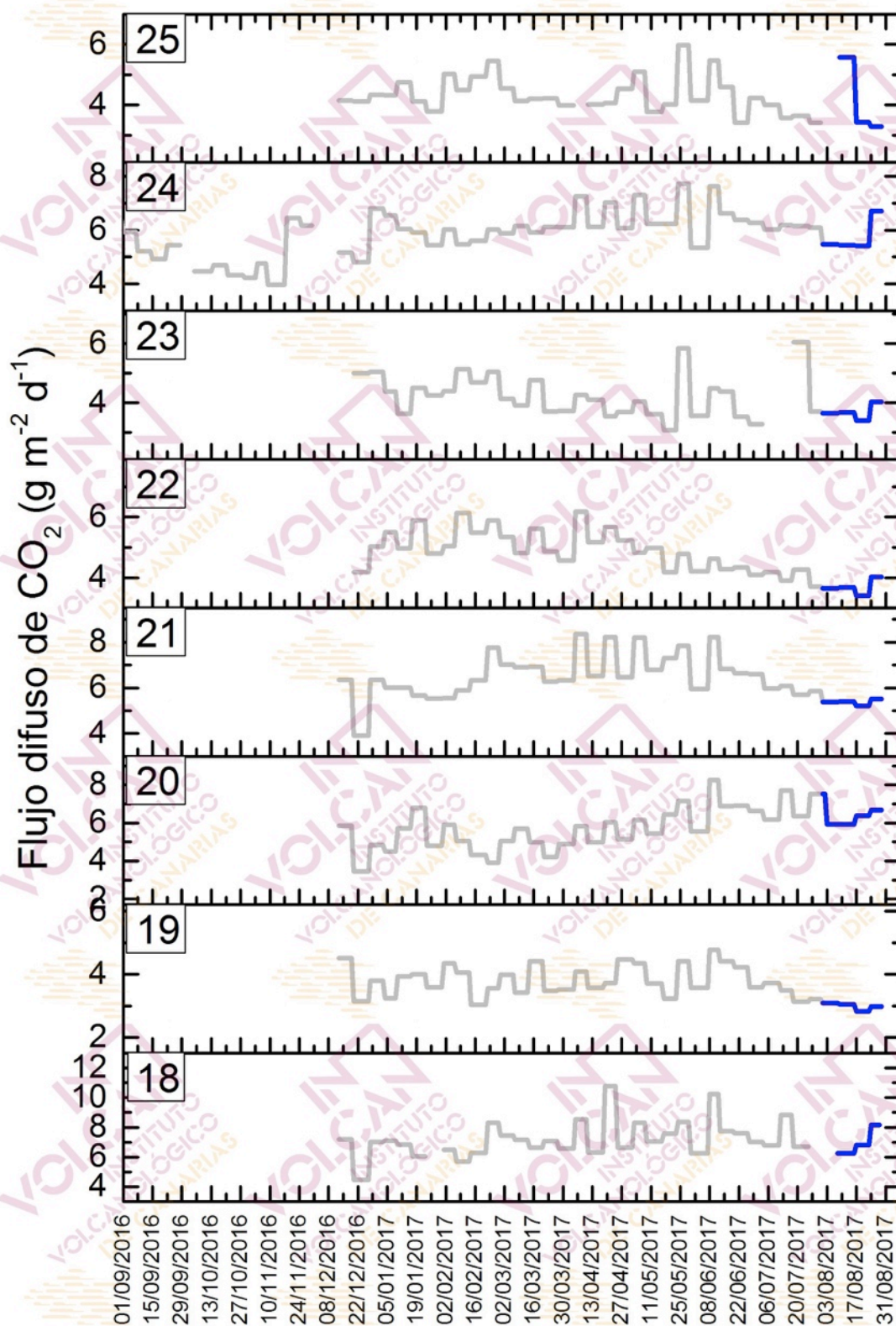
Figura 4.7 – Monitorización semanal del flujo difuso de CO 2 en la Red de Trampas Alcalinas de la Caldera de Las Cañadas principalmente desde diciembre de 2016. Los datos de agosto de 2017 se encuentran marcados en azul oscuro.
