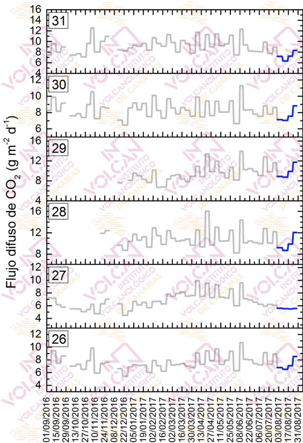
Figura 4.5 – Monitorización semanal del flujo difuso de CO 2 en la Red de Trampas Alcalinas del sistema volcánico Dorsal Noreste de Tenerife desde septiembre de 2016. Los datos de agosto de 2017 se encuentran marcados en azul oscuro.
