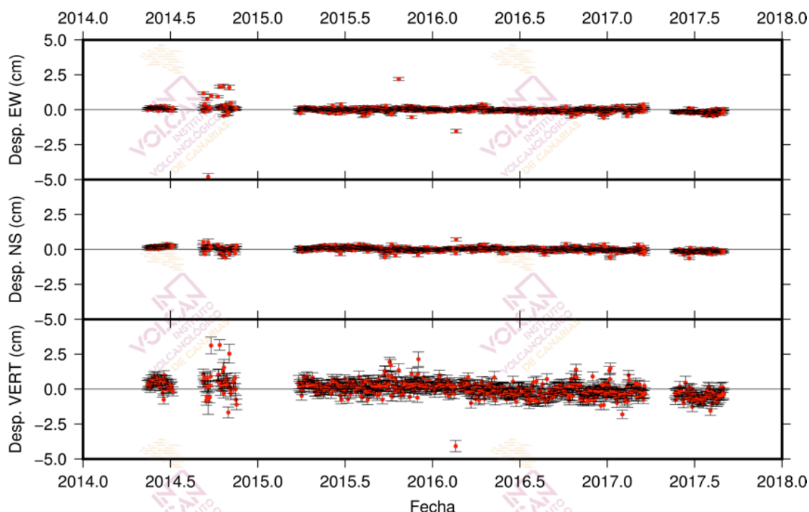
Figura 3.2 – Series temporales de los desplazamientos verticales y horizontales registrados por la estación GPS IZAN (Izaña) desde 2014. El valor medio y la incertidumbre para cada día se indican en rojo y negro, respectivamente.
