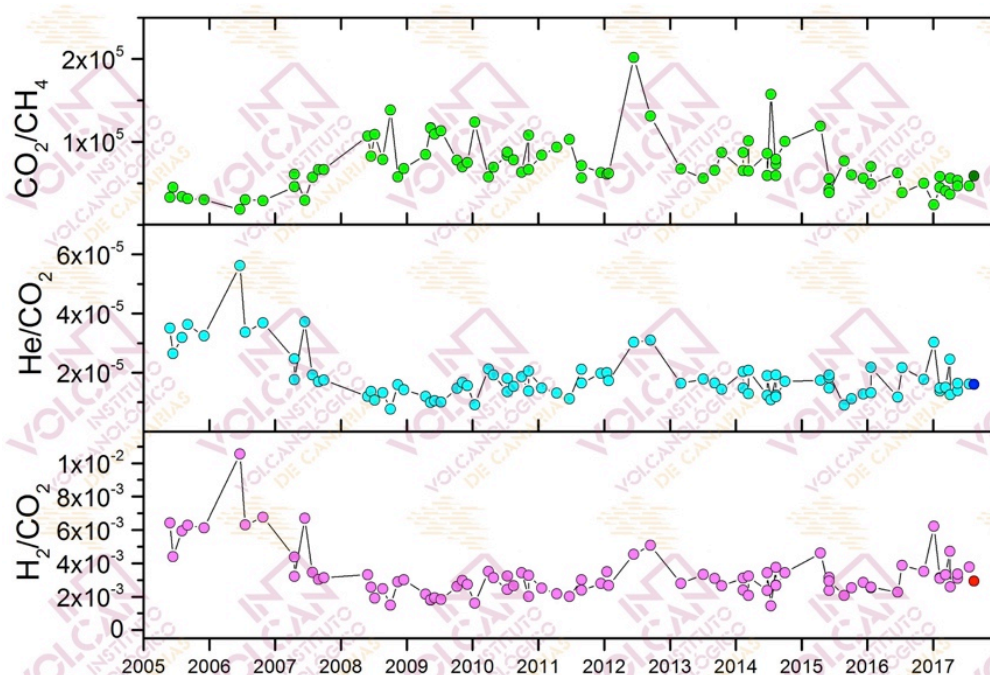
Figura 4.8 - Variaciones temporales de las relaciones molares \text{CO}_2/\text{CH}_4 , \text{He}/\text{CO}_2 y \text{H}_2/\text{CO}_2 en las fumarolas del Teide (TEF1). Los datos de agosto de 2017 se encuentran indicados en diferentes colores.
