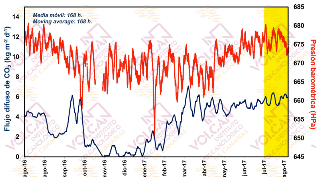
Figura 4.2 - Monitorización de la media móvil semanal del registro en modo continuo del flujo de CO 2 (azul) y la presión barométrica (rojo) de la estación geoquímica TFG12 (Mirador de la Fortaleza del Teide, Tenerife). Los datos de julio y agosto de 2017 se encuentran indicados por el área amarilla.
