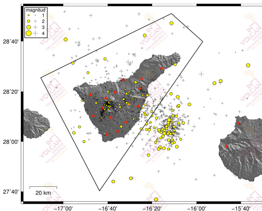
Figura 1.1 - Hipocentros de los terremotos localizados por la Red Sísmica Canaria (triángulos rojos) en agosto de 2017 (círculos amarillos). Las cruces muestran los hipocentros localizados en los últimos 12 meses. El polígono negro corresponde al área de Tenerife considerada para las estadísticas sismológicas en los gráficos siguientes. [La fuente de los datos sísmicos anteriores al 21/11/2016 es el Instituto Geográfico Nacional, IGN].
