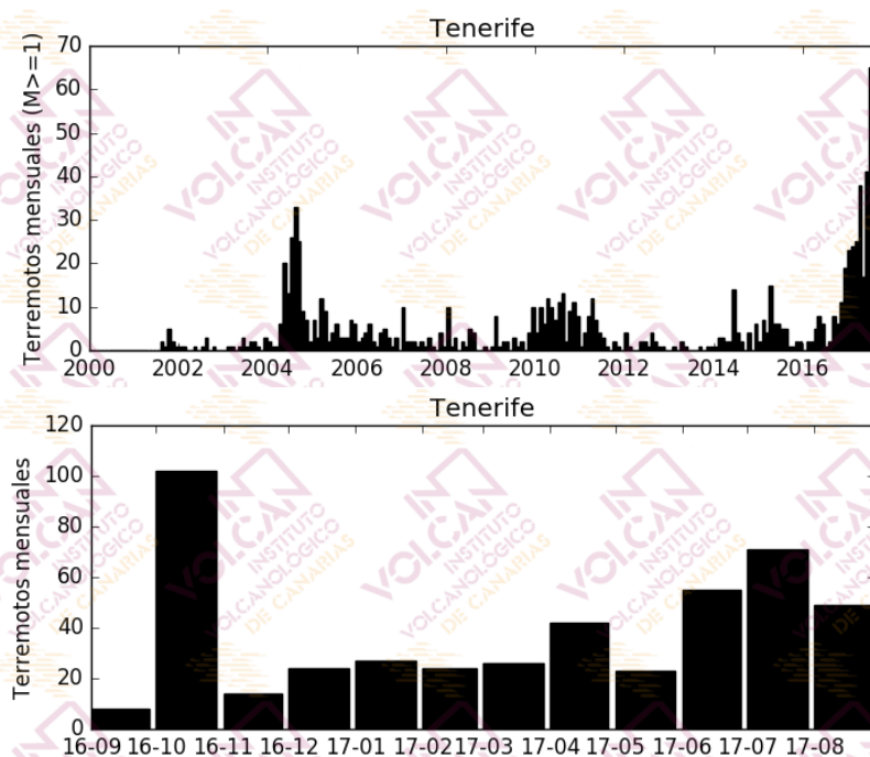
Figura 1.2 - Número de terremotos mensuales en Tenerife. El histograma superior corresponde al periodo enero 2000-agosto 2017 para terremotos con M \geq 1 , mientras que el inferior muestra el periodo septiembre 2016-agosto 2017 para todas las magnitudes. [La fuente de los datos sísmicos anteriores al 21/11/2016 es el Instituto Geográfico Nacional, IGN].
