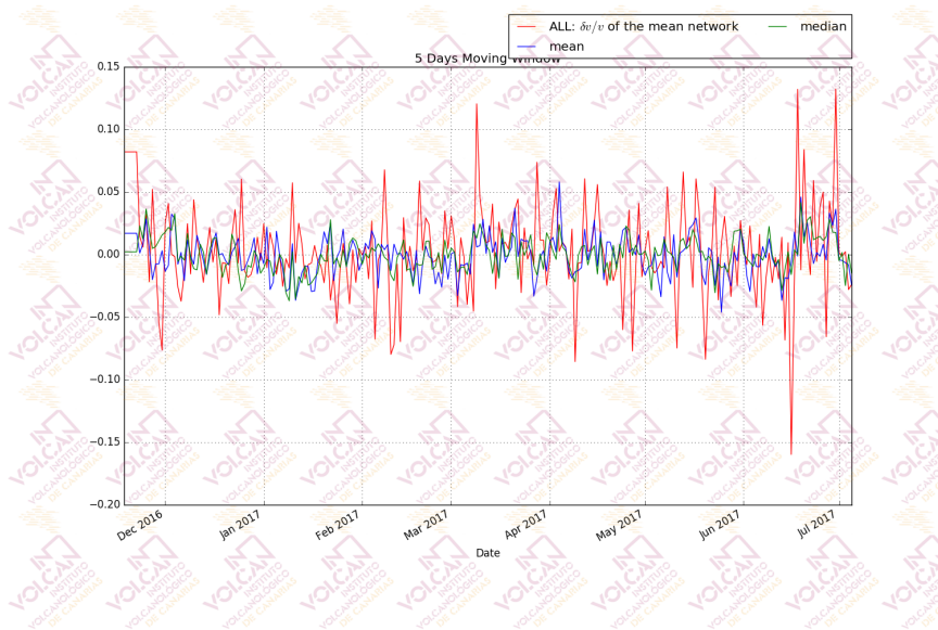
Figura 1.7 - Variaciones de velocidad relativa (% dv/v ) medidas por interferometría sísmica (software MSNoise) desde noviembre 2016 hasta agosto 2017.
