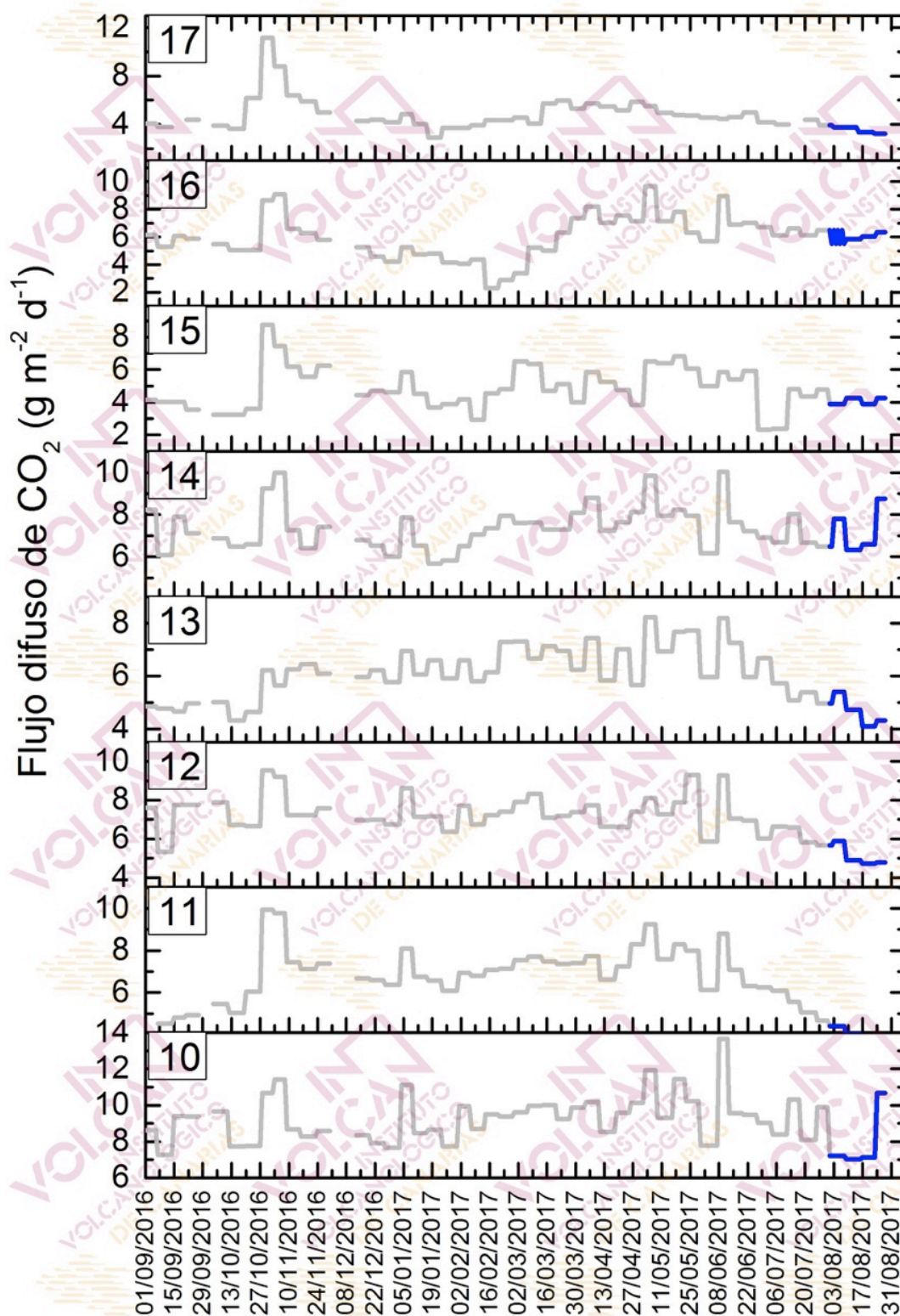
Figura 4.6 – Monitorización semanal del flujo difuso de CO 2 en la Red de Trampas Alcalinas del sistema volcánico Dorsal Norte-Sur de Tenerife desde septiembre de 2016. Los datos de agosto de 2017 se encuentran marcados en azul oscuro.
