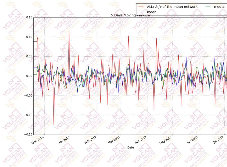
Figura 1.7 - Variaciones de velocidad relativa (% dv/v ) medidas por interferometría sísmica (software MSNoise) desde noviembre 2016 hasta julio 2017.
